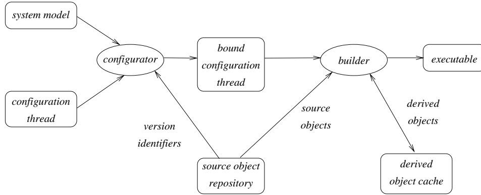
Fig. 22. DSEE.
