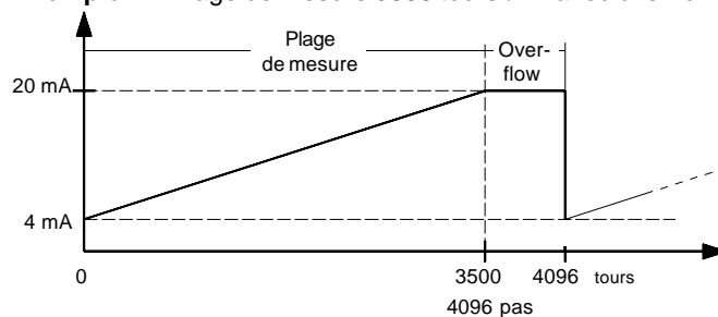
Exemple 4 : Plage de mesure 3500 tours ≠ 2 n avec overflow
