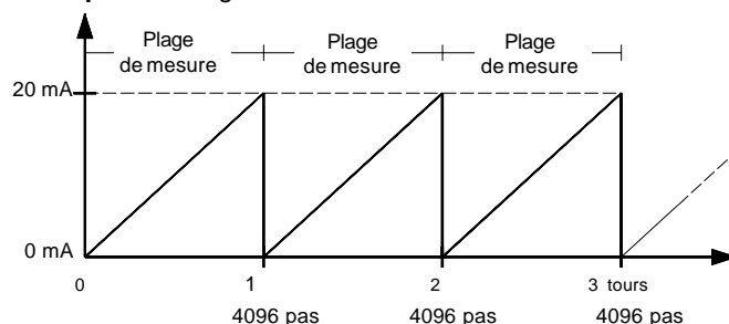
Exemple 2 : Plage de mesure 1 tour = 2 n
