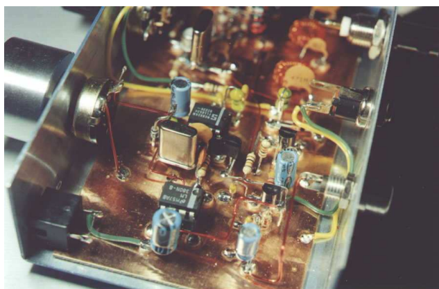
TT2/MRX Combo.
