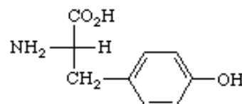
Tyrosine
