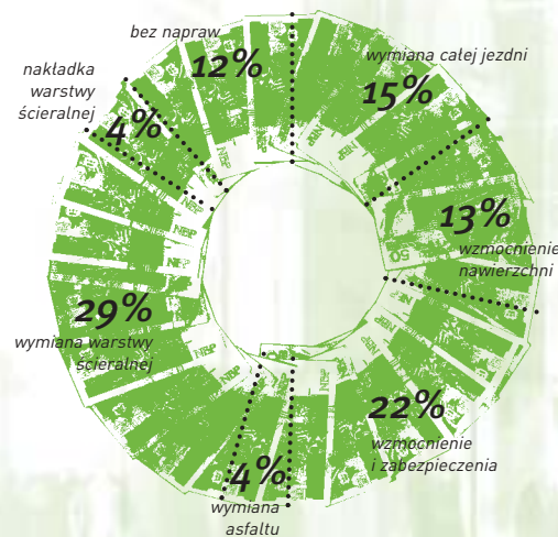
Wykres 12. Zakres niezbędnych napraw dróg w Warszawie w 2003 roku
