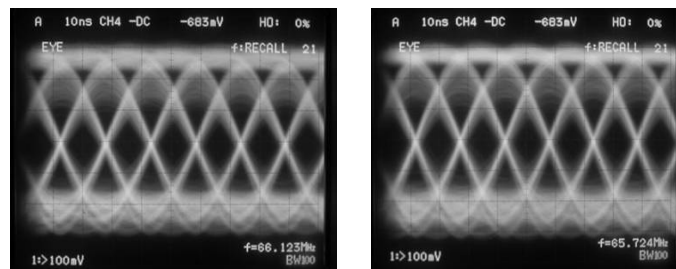
Layer 0 Layer 1 Jitter 5.6 % Jitter 5.8 % (Limit-Equalizer)
