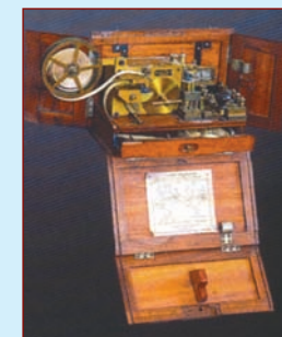
Облегченный кавалерийский телеграфный аппарат 1914 г.
