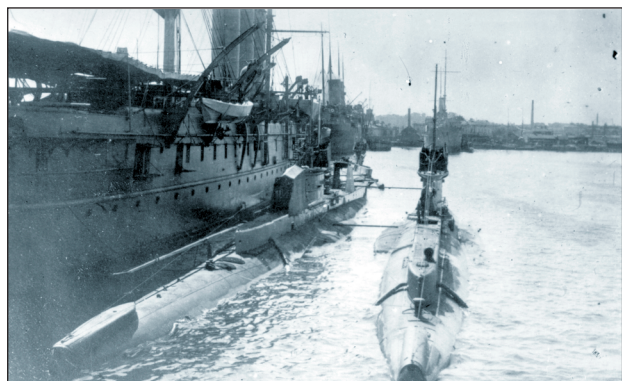
Английские подводные лодки типа «Е» у борта плавбазы «Двина» в Ревеле
