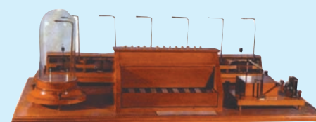
Телеграфный аппарат Шиллинга
