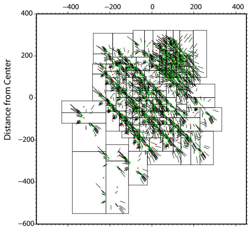
Layer 9 (215–285 km)
