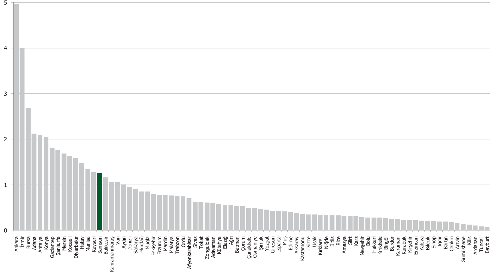
Grafik 1.5 Nüfus, 2012
