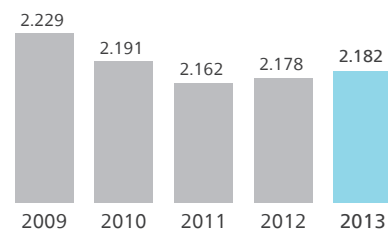
Consumo specifico netto della produzione termoelettrica semplice (kcal/kWh)
