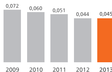
Emissioni specifiche di polveri della produzione termoelettrica semplice (g/kWh termo netto)
