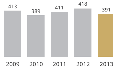
Emissioni specifiche di CO 2 della produzione termoelettrica semplice e combinata riferite alla produzione complessiva di energia elettrica e calore (g/kWh totale netto)
