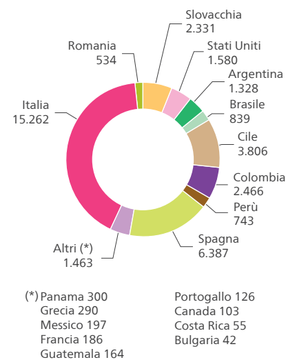
Parco di generazione rinnovabile al 31.12.2013 Totale: 36.739 MW
