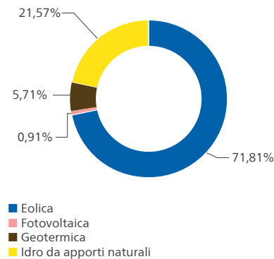
Produzione netta di energia elettrica Totale: 4.913 milioni di kWh
