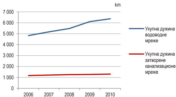
Графикон 12.2. Укупна дужина водоводне и канализационе мреже
