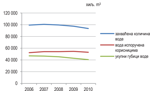
Графикон 12.1. Захваћена и испоручена вода, губици воде
