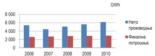
14.1. Нето производња и финална потрошња електричне енергије
