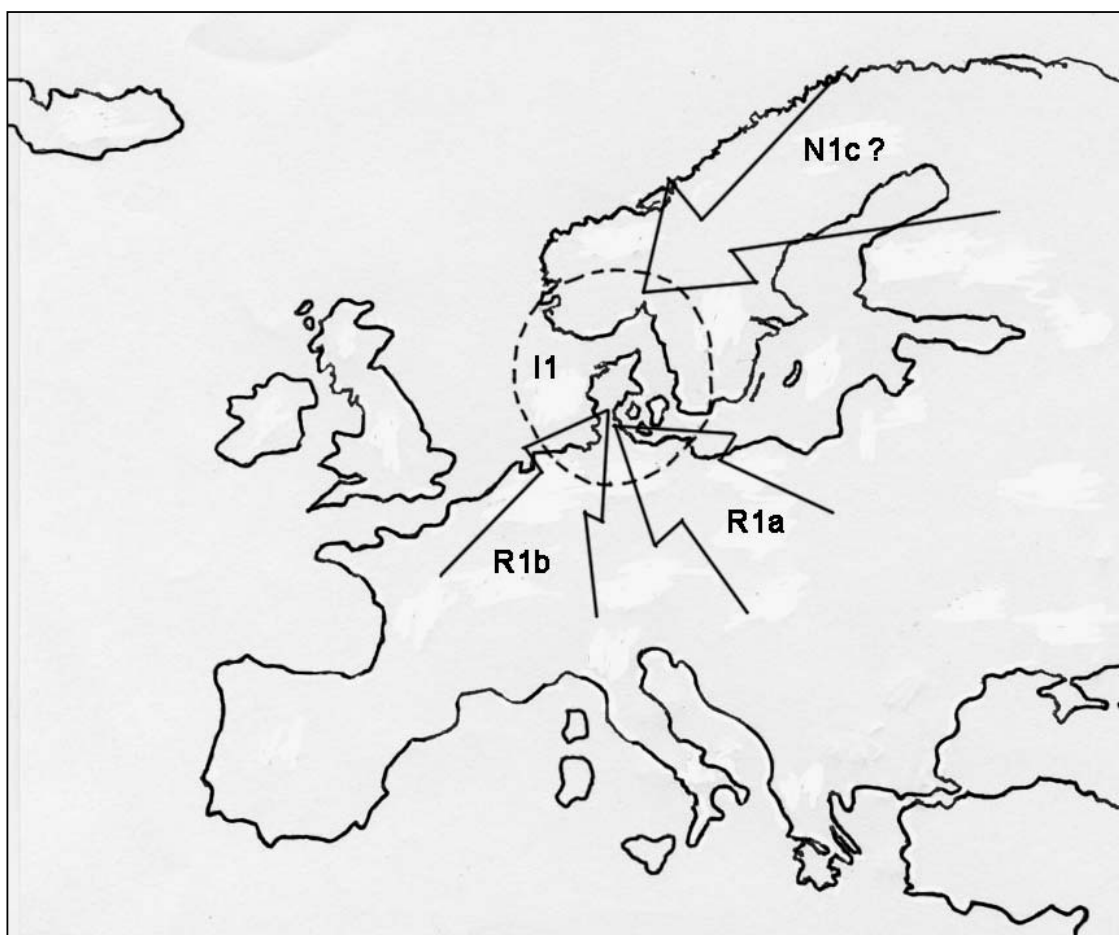
Рис. 15. Распространение хромосомных гаплогрупп в 3000–1000 гг. до н. э.
