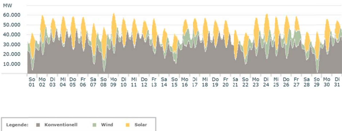
Abbildung 58: Simuliertes Last- und Stromerzeugungsprofil auf Basis beispielhafter Wetterdaten für eine sonnige Maiwoche bei installierten Leistungen von 50 GW PV und 40 GW Wind, die Spitzenleistungen von 35 GW PV und 21 GW Wind liefern (B. Burger, Fraunhofer ISE)
