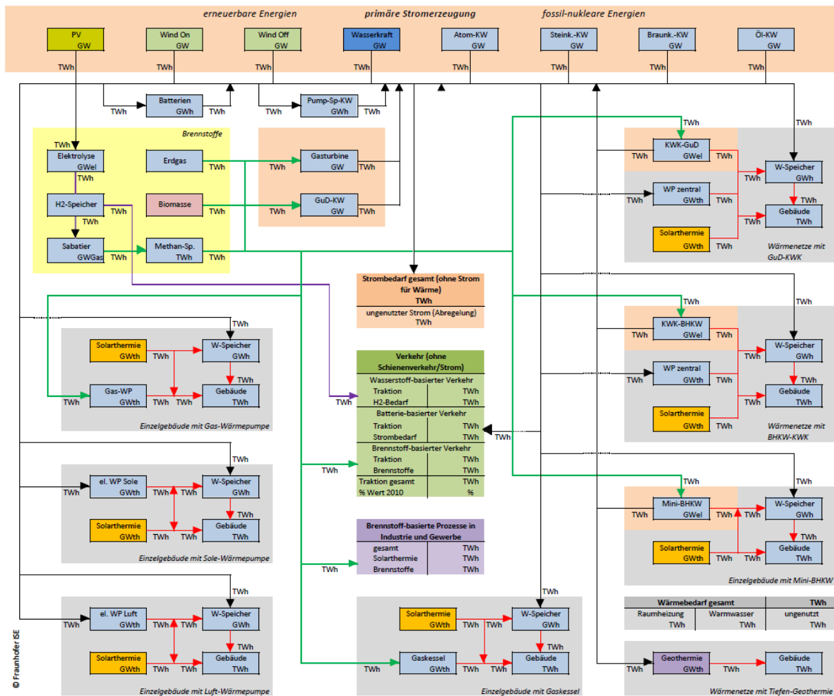
Abbildung 47: Szenario eines deutschen Energiesystems, schematische Darstellung der Systemzusammensetzung. [ISE5]
