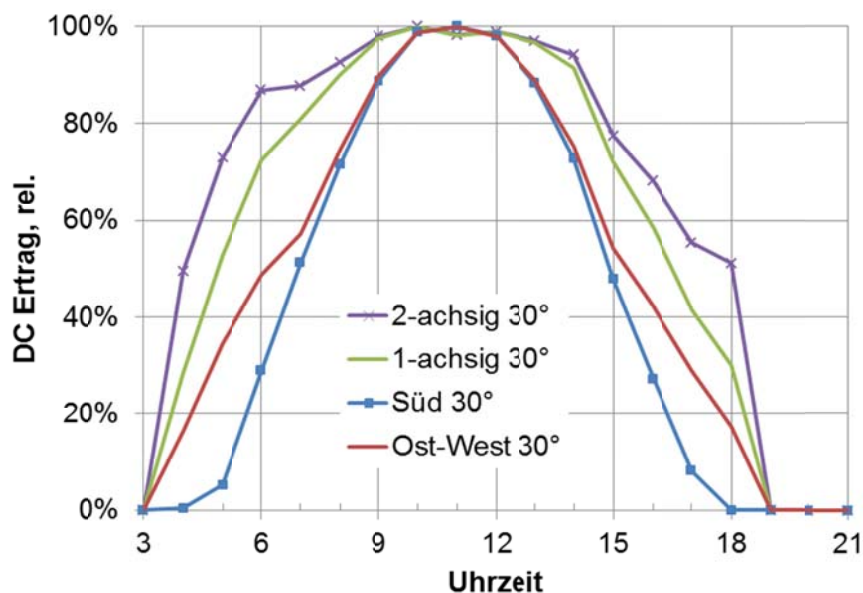
Abbildung 59: Stromertragsprofile von PV-Anlagen in verschiedenen Montagevarianten, berechnet mit der Software PVsol für einen überwiegend klaren Julitag am Standort Freiburg
