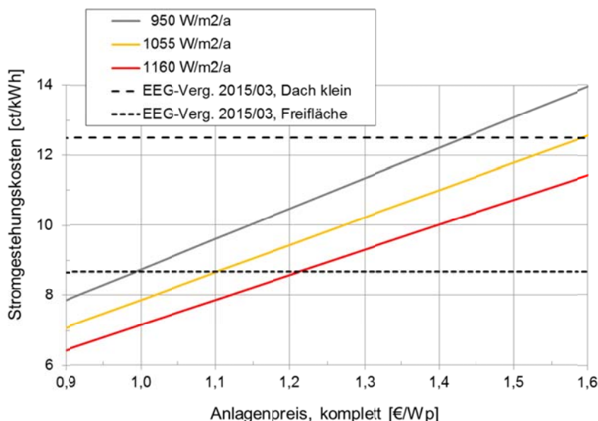
Abbildung 27: Grobe Abschätzung der Stromgestehungskosten für PV-Anlagen unter verschiedenen Einstrahlungsbedingungen
