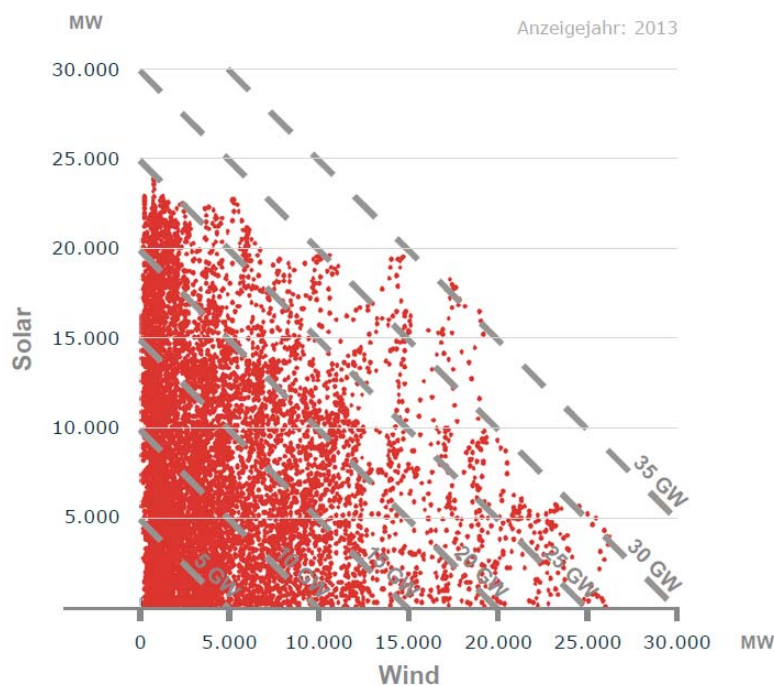
Abbildung 34: Mittlere Stundenleistung für die Einspeisung von Sonnen- und Windstrom im Jahr 2013 [ISE4]
