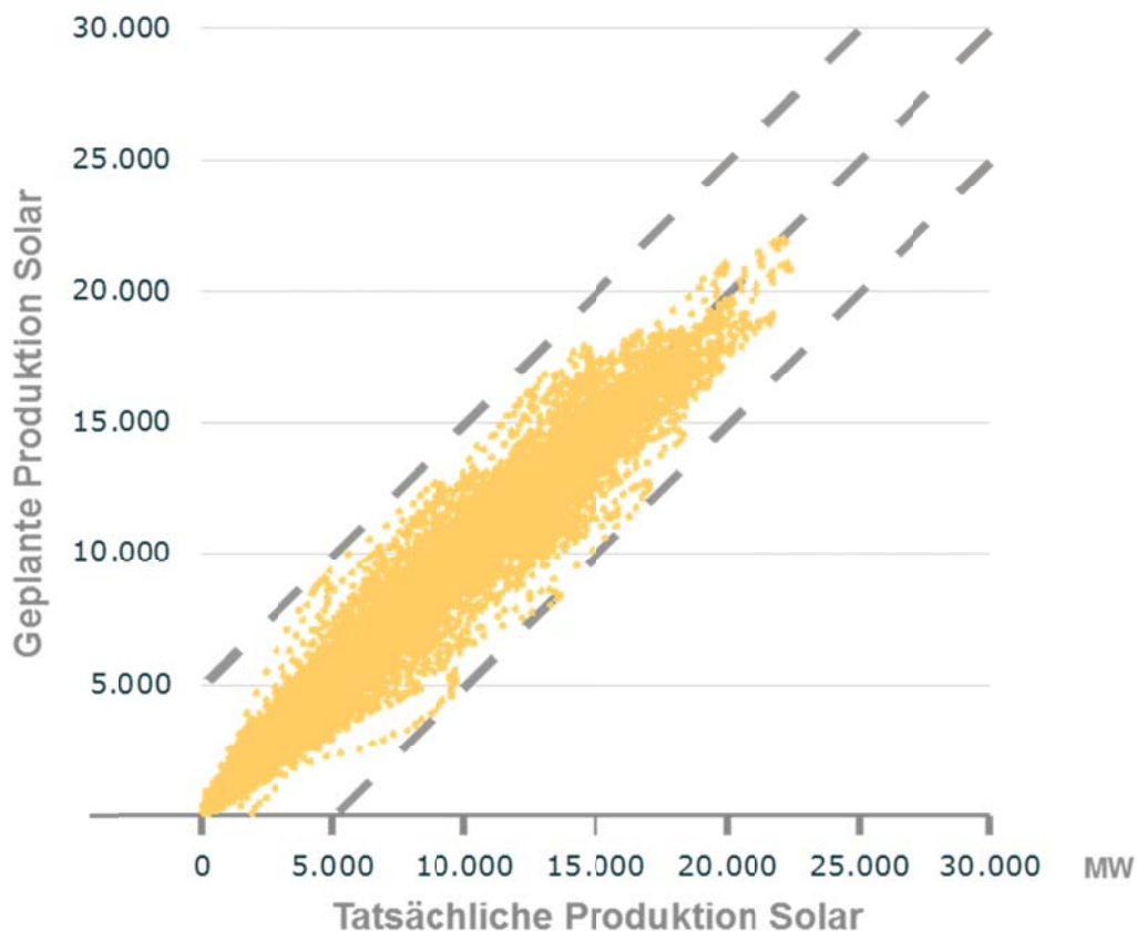
Abbildung 33: Stündliche tatsächliche und geplante Stromproduktion im Jahr 2012 [ISE4]
