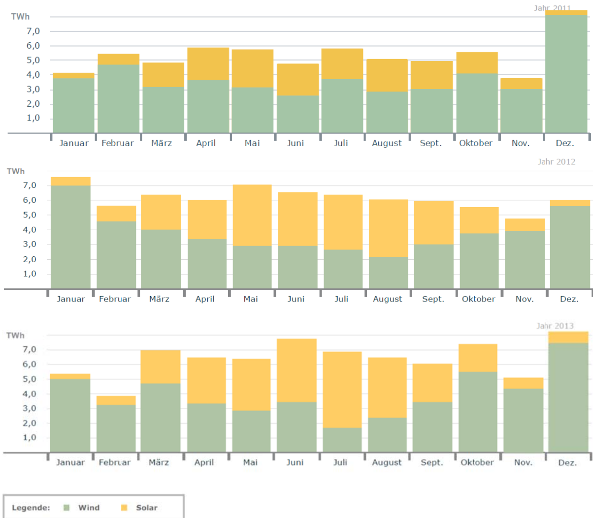
Abbildung 35: Monatliche PV- und Windstromproduktion der Jahre 2011-2013 [ISE4]
