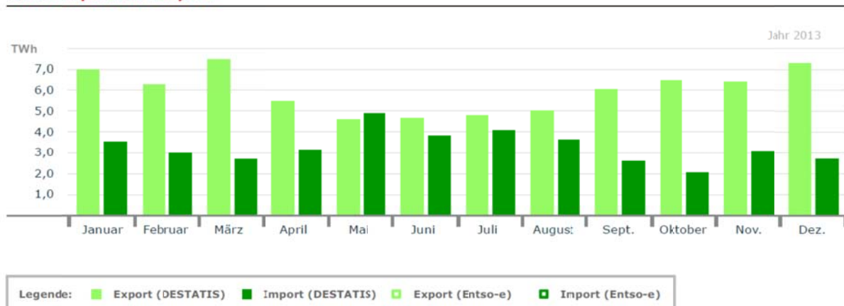
Abbildung 26: Monatliche Export- und Importmengen im Jahr 2013 [ISE4]
