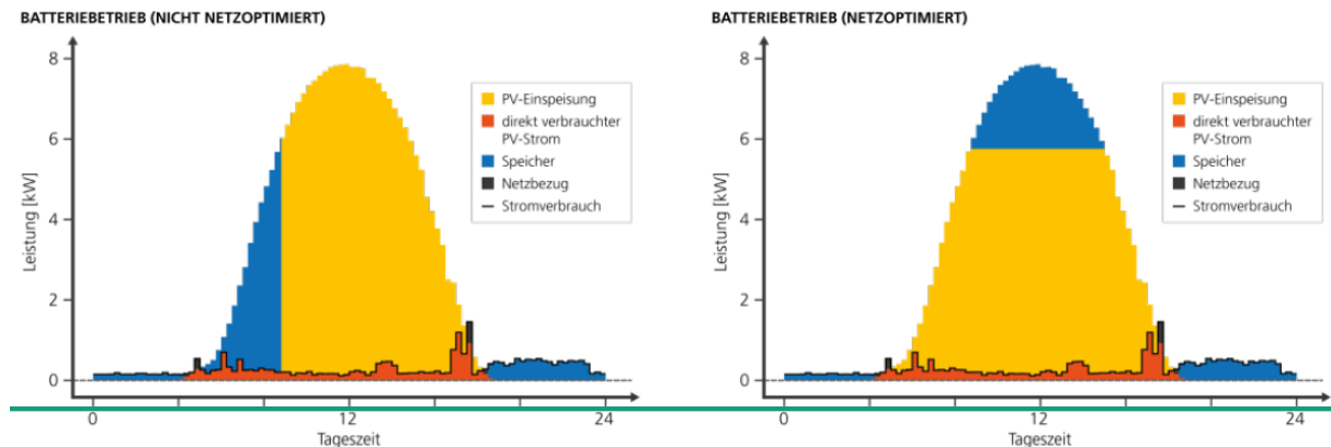
Abbildung 64: Gegenüberstellung der konventionellen und der netzdienlichen Betriebsführung [ISE7]
