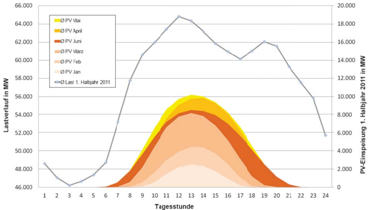
Abbildung 57: Durchschnittliches Lastprofil und durchschnittliche monatliche PV-Einspeisepprofile im ersten Halbjahr 2011 [IZES]
