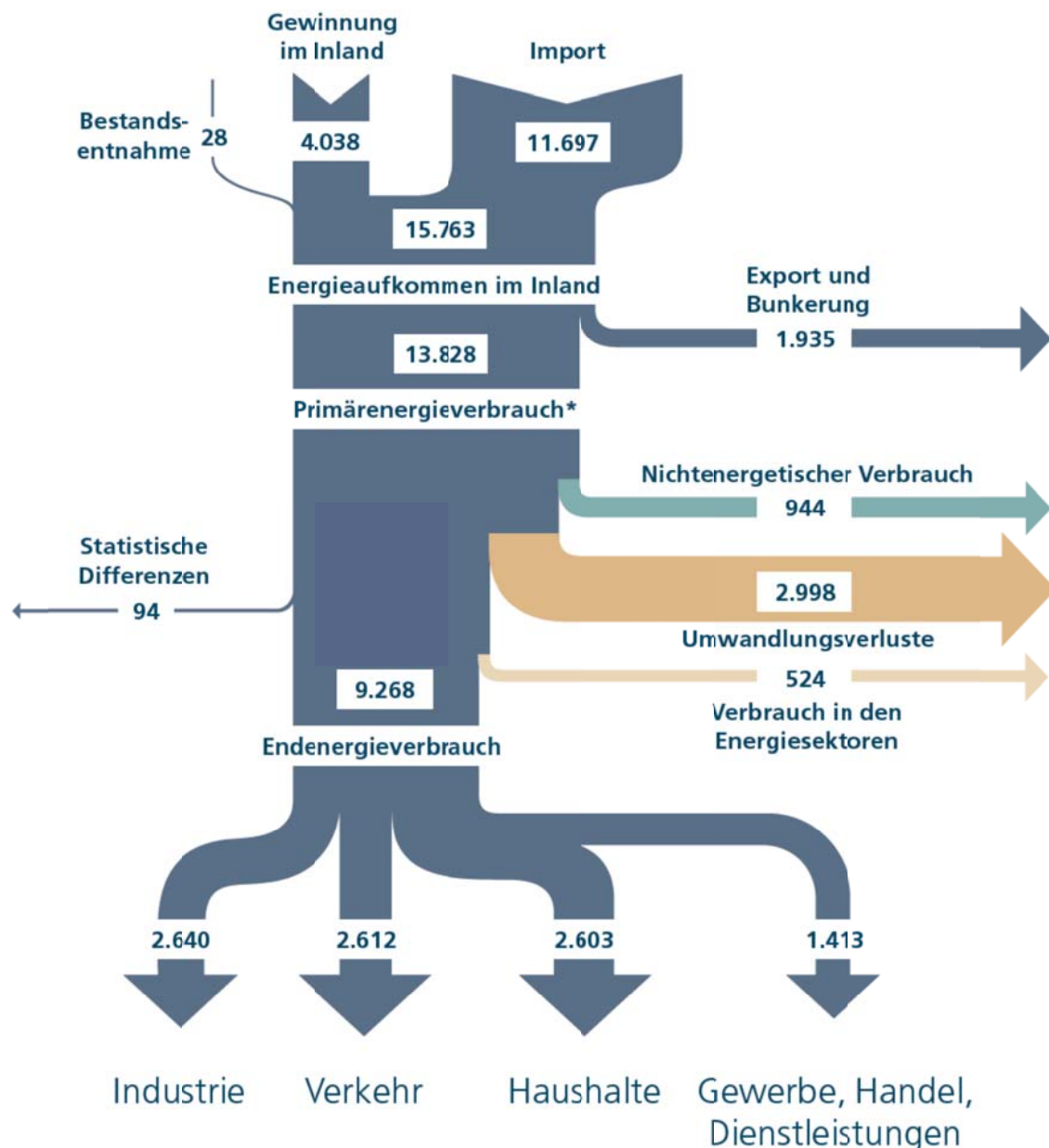
Abbildung 50: Energieflussbild 2013 für Deutschland, Angaben in Petajoule, Zahlen vorläufig/geschätzt [AGEB2]
