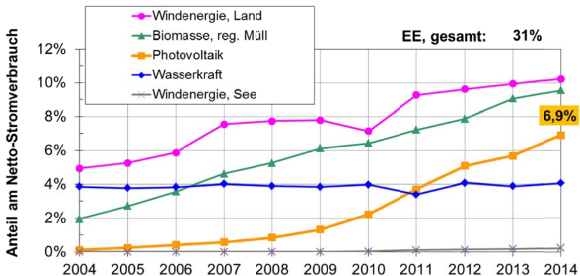
Abbildung 1: Entwicklung des Anteils Erneuerbarer Energien am Netto-Stromverbrauch (Endenergie) in Deutschland, Daten aus [BMW1], [AGEB5], [AGEB6], Pressemitteilung BDEW
