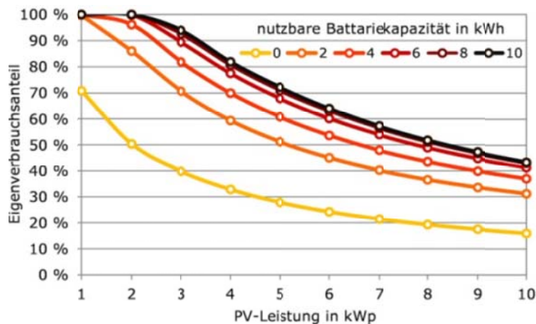
Abbildung 63: Eigenverbrauchsanteil in Abhängigkeit von Batteriekapazität und Leistung des Solargenerators für einen Einfamilienhaushalt mit einem Jahresstromverbrauch von 4.700 kWh. [Quasch]
