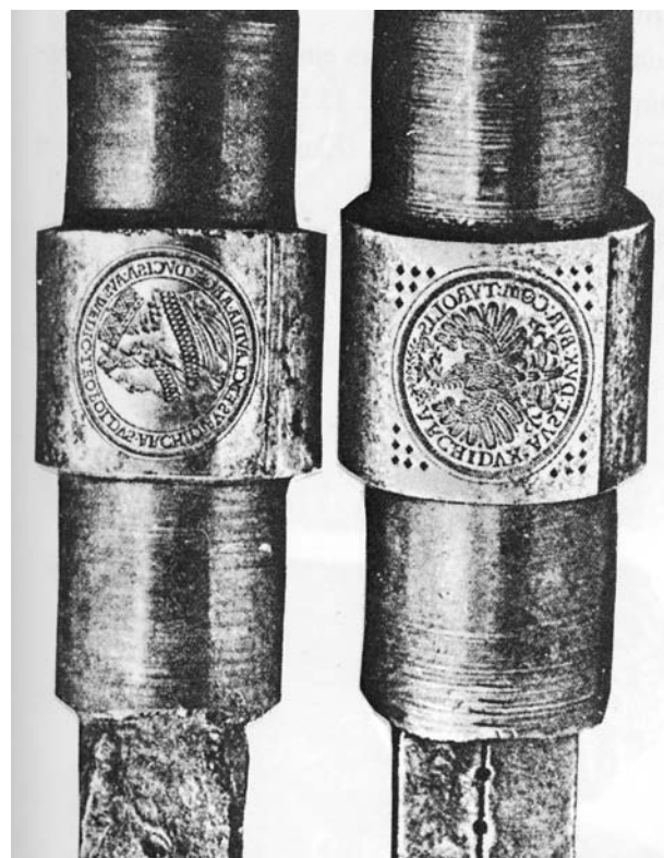
Bild 4: Graviertes Walzenpaar.
