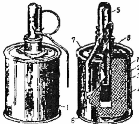
Рис. 21. Граната РГ-42
