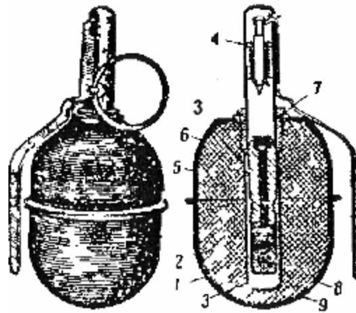
Рис. 22. Граната РГД-5
