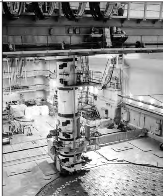
Ленинградская АЭС
