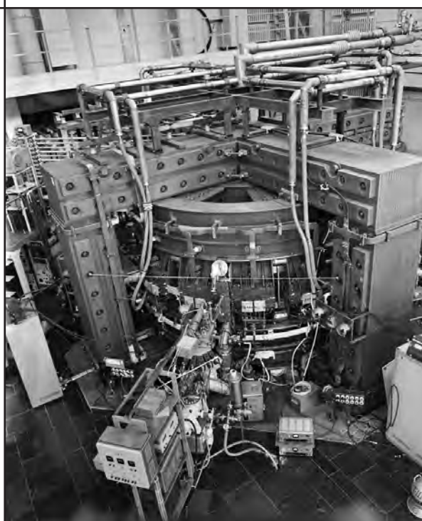
Токамак Т-10
