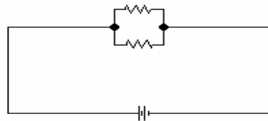
Fig. 5: Resistencias en paralelo
