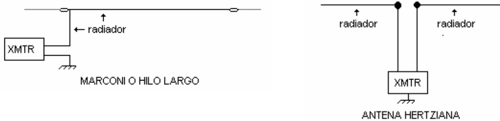
Fig. 24: Antenas Marconi y Hertziana
