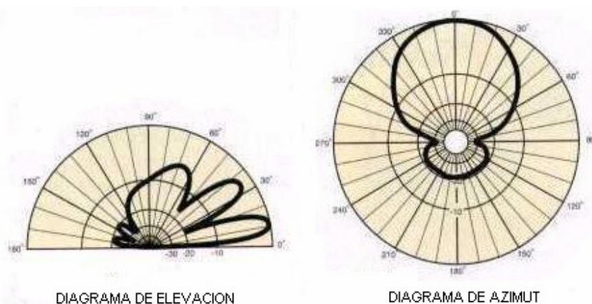
Fig. 23: Diagramas de radiación en elevación y de azimut
