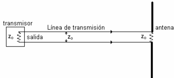
Fig. 20: Impedancia característica
