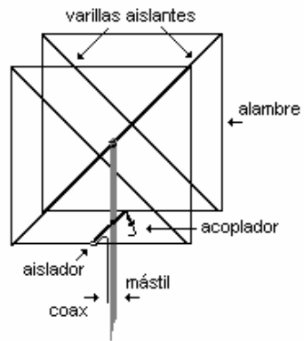
Fig. 34: Antena cuadracúbica
