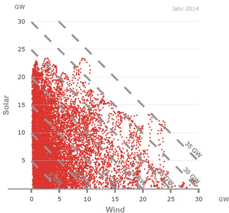
Abbildung 28: Mittlere Stundenleistung für die Einspeisung von Sonnen- und Windstrom im Jahr 2014 [ISE4]
