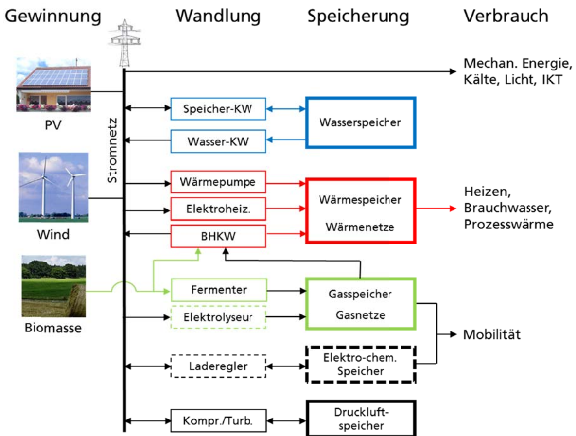
Abbildung 39: Vereinfachte schematische Darstellung eines Erneuerbaren Energiesystems mit den wichtigsten stromnetzgebundenen Bausteinen der Kategorien Gewinnung, Wandlung, Speicherung und Verbrauch; IKT: Informations- und Kommunikationstechnik; gestrichelte Kästen: zur Zeit noch sehr geringe Leistungen/Kapazitäten verfügbar
