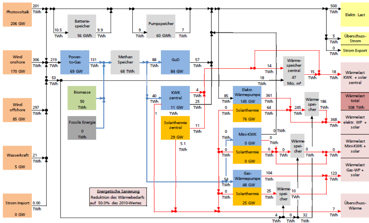
Abbildung 41: Szenario eines deutschen Energiesystems, schematische Darstellung der Systemzusammensetzung. [ISE5]
