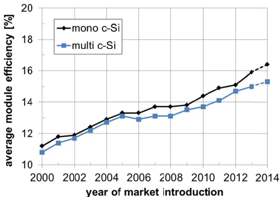
Abbildung 31: Entwicklung der mittleren Wirkungsgrade von PV-Module auf Basis von mono- und multikristallinen Zellen nach dem Jahr der Markteinführung, Daten aus Photon International 2014-02
