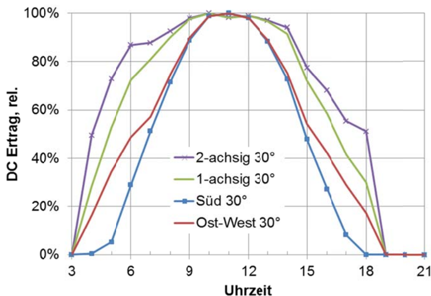
Abbildung 53: Stromertragsprofile von PV-Anlagen in verschiedenen Montagevarianten, berechnet mit der Software PVsol für einen überwiegend klaren Julitag am Standort Freiburg
