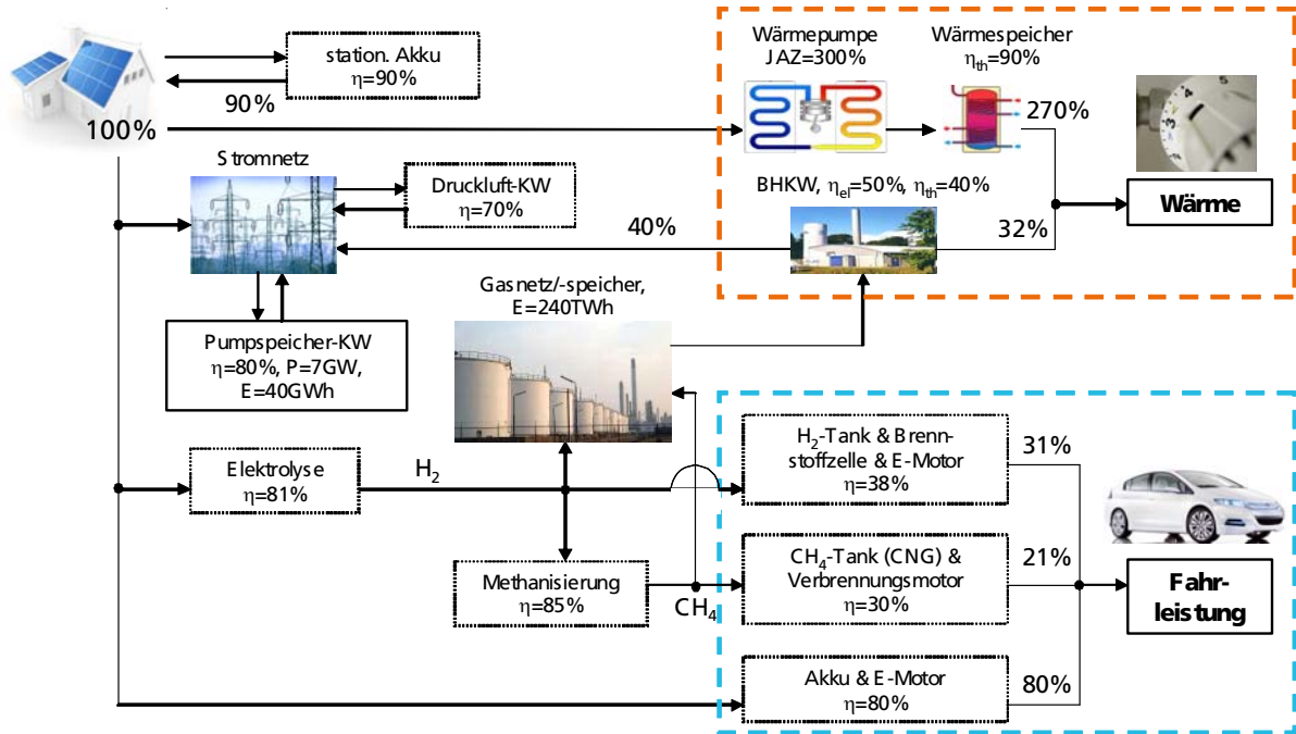
Abbildung 59: Mögliche Pfade zur Wandlung und Speicherung von PV-Strom mit orientierenden Angaben zu Wirkungsgraden
