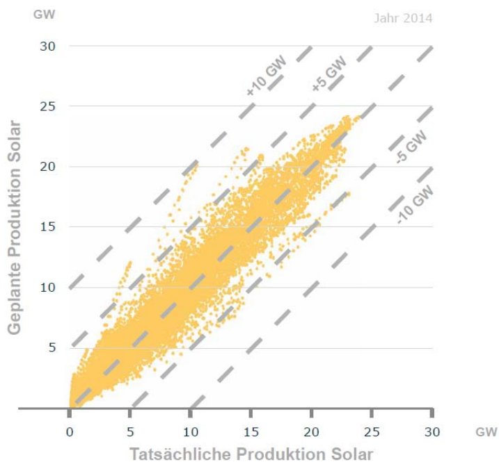
Abbildung 27: Stündliche tatsächliche und geplante Stromproduktion im Jahr 2014 [ISE4]
