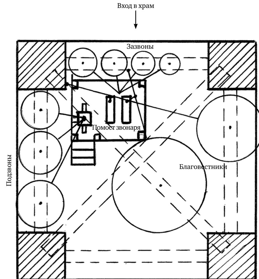
Вариант правильного размещения колоколов и тяг для управления ими в храме «Иже под колоколы» (квадратный ярус звона). Схема предоставлена Московским колокольным центром
