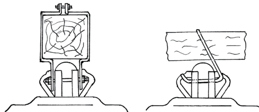
Рис. 3. Фиксация крепежного хомута на балке
