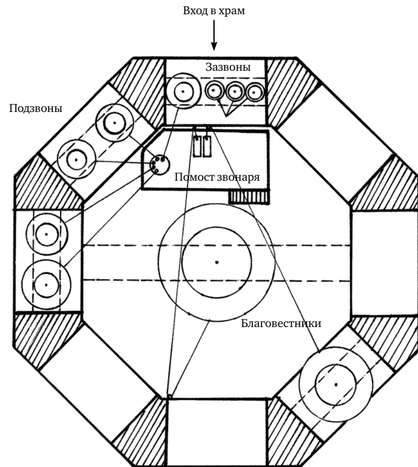
Вариант правильного размещения колоколов и тяг для управления ими в храме «Иже под колоколы» (восьмигранный шатер). Схема предоставлена Московским колокольным центром
