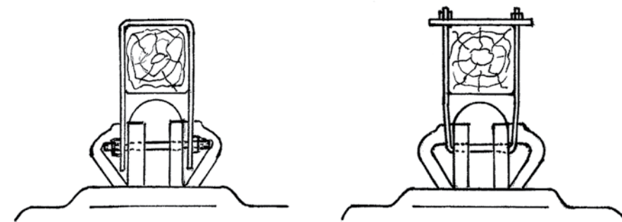
Рис. 2. Пропуск опорной шпильки в сквозные отверстия хомутов и уши колокола
