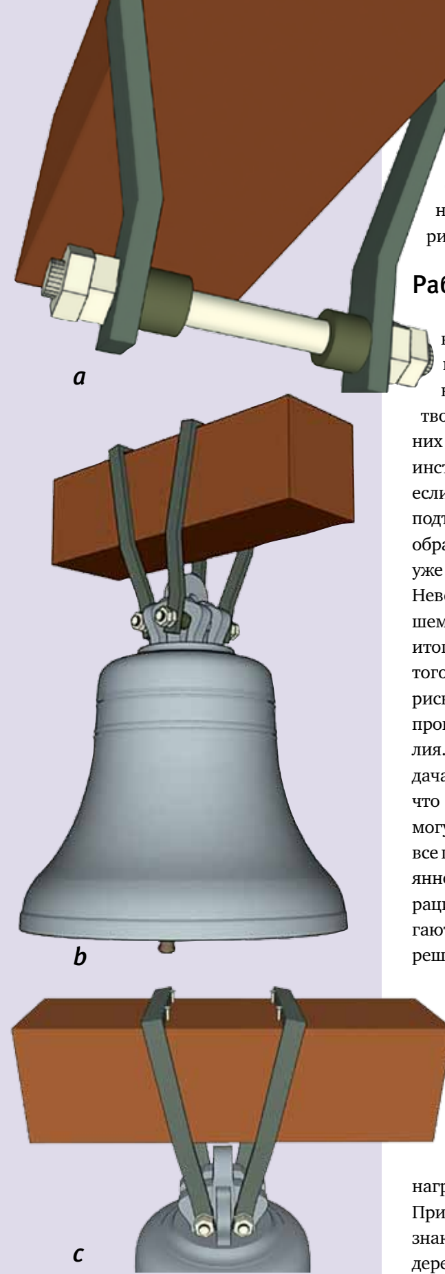
Финальный этап закрепления колокола на несущей балке: подготовка опорной шпильки (а), подвес колокола (b), фиксация хомутов (с) (чертежи Общества церковных звонарей)
