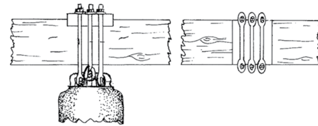
Рис. 1. Правильная установка хомутов на балку
