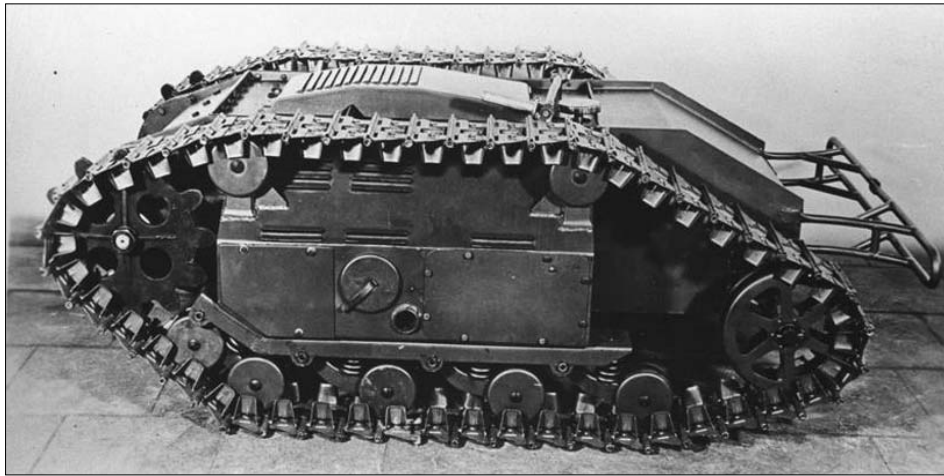
„Goliat” - samobieżna mina na gąsienicach napędzana własnym silnikiem spalinowym, sterowana za pomocą kabla elektrycznego
