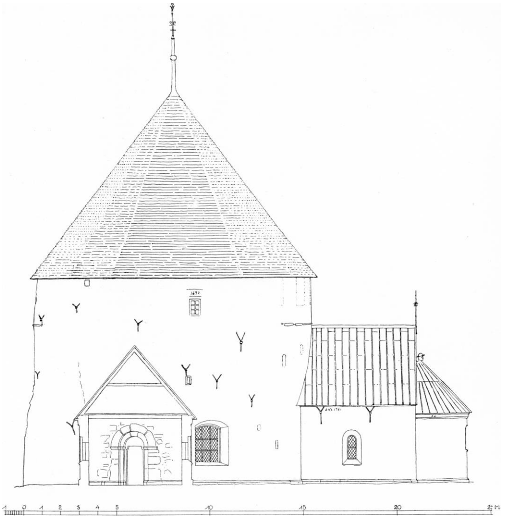
Fig. 6. Nylars kirke, set fra syd. 1:200. Målt af Charles Christensen 1939.
