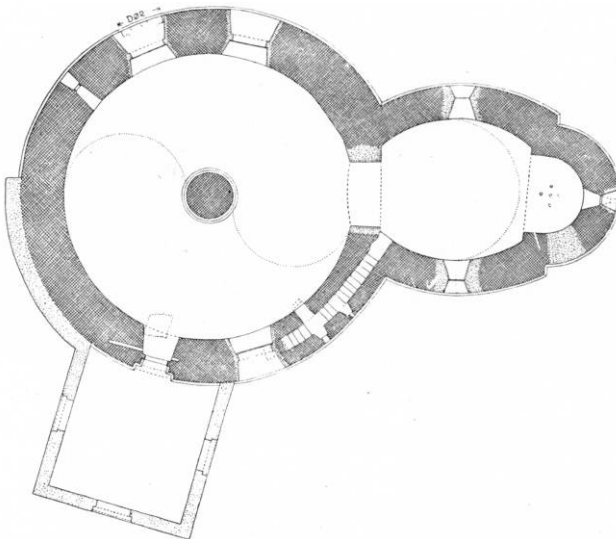
Fig. 2. Nylars kirke. Grundplaner, 1:300. Målt af Charles Christensen 1939.
