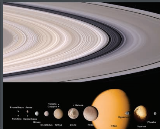
Einige Monde des Saturn
