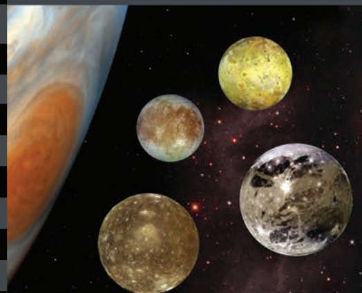
Die "Galileischen Monde" des Jupiter
