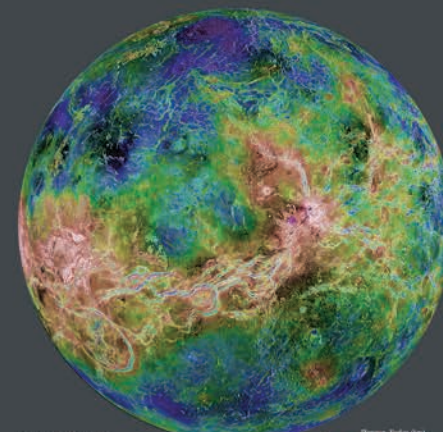
Venus Relief Falschfarbendarstellung der östlichen Hemisphäre
