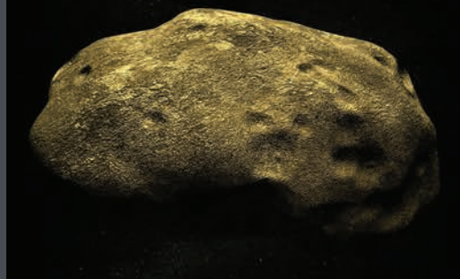
Asteroiden sind meist unregelmäßig geformt. Nur wenn die Masse und damit die Schwerkraft groß genug ist, bildet sich eine kugelförmige Gestalt.
