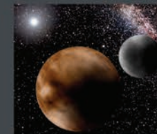
Pluto und Charon
