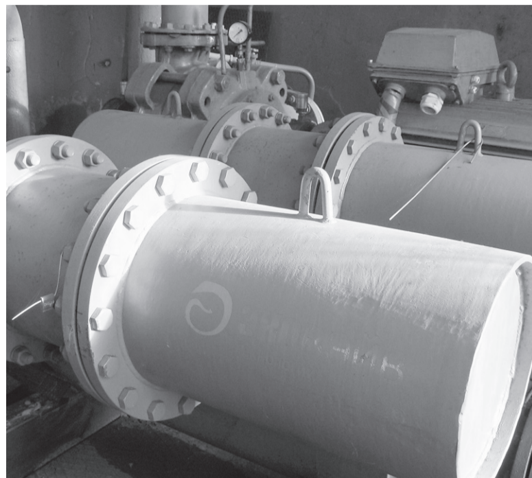
Установка стабилизаторов давления в МУП г. Ижевска «Ижводоканал».
