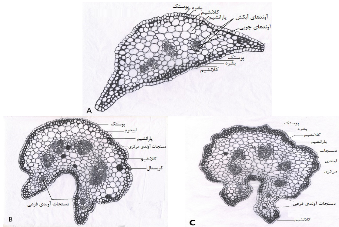
شکل ۵: انواع دمبرگ در جنس A. Amaranthus : A: دمبرگ در A. albus (طرح رسم شده از عکس ۳A) تعداد لایه های کلانشیم و پارانشیم کم و فاقد دستجات آوندی فرعی، B: دمبرگ در A. hybridus (طرح رسم شده از عکس ۳H) و C: دمبرگ در A. tricolor (طرح رسم شده از عکس ۳E) لایه های کلانشیم و پارانشیم بیشتر و دارای دستجات آوندی فرعی.
