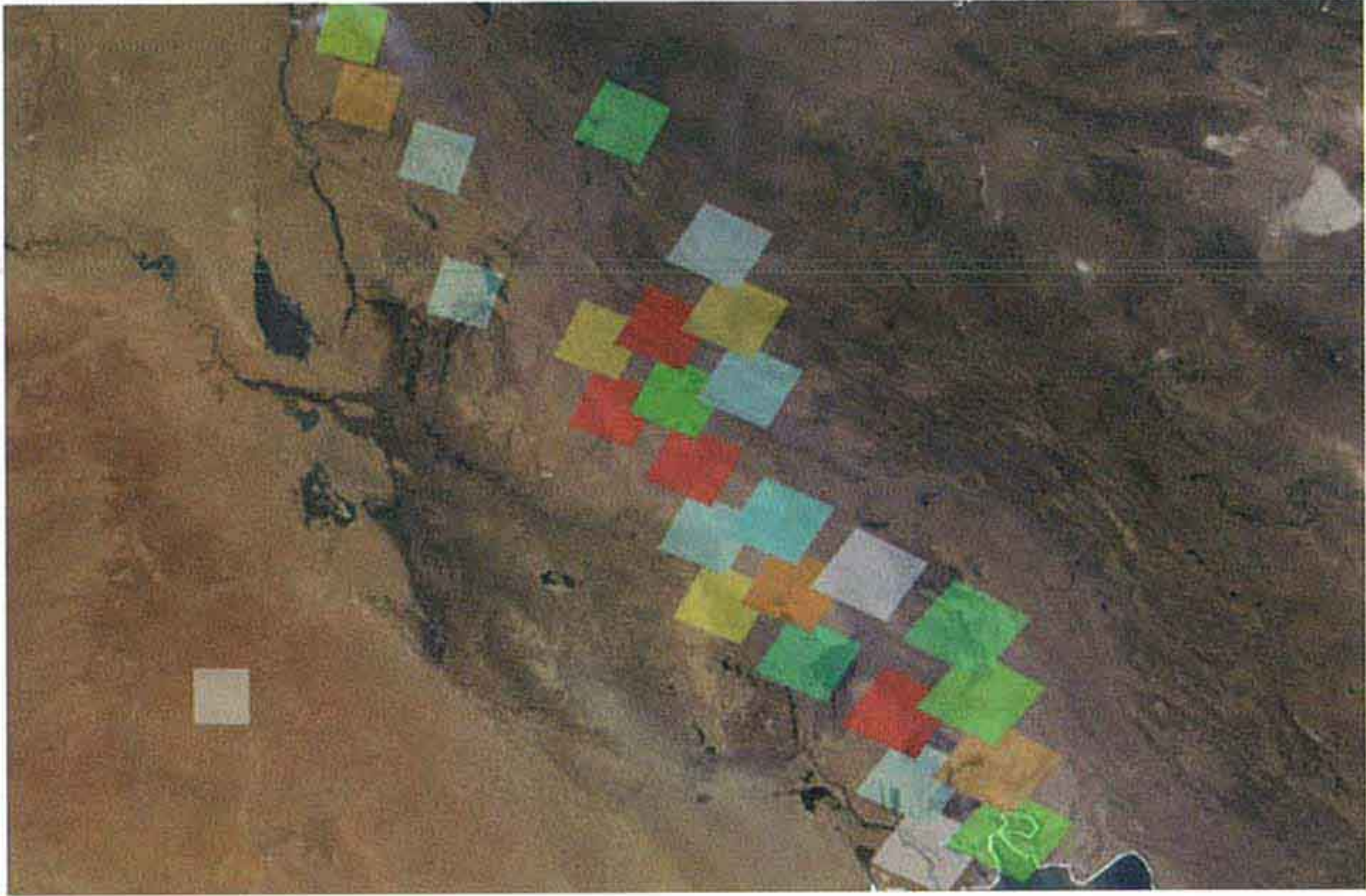
صورة فضائية لمنطقة في ٢٥ يونيو ٢٠٠٣ لأدخنة مصنع الكبريت المحترق في جنوب العراق
