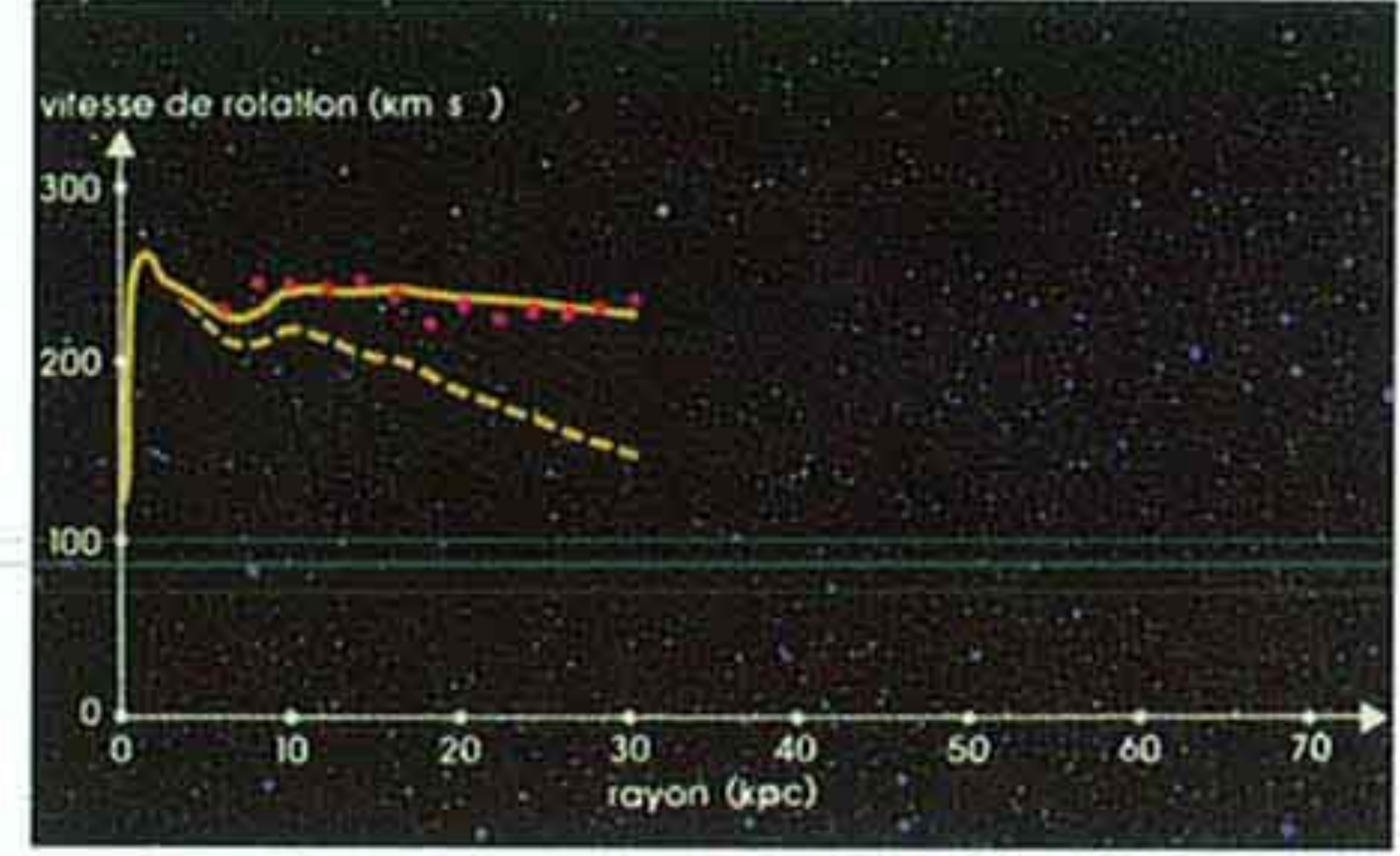
تباين سرعة دوران النجوم المتوقعة (المنحنى المنقطع) والمقاسة فعلاً (المنحنى المنقط) مقدرة كم/ثا مع بعد المسافة عن مركز المجرة مقدراً بالكيلوبارسيك
