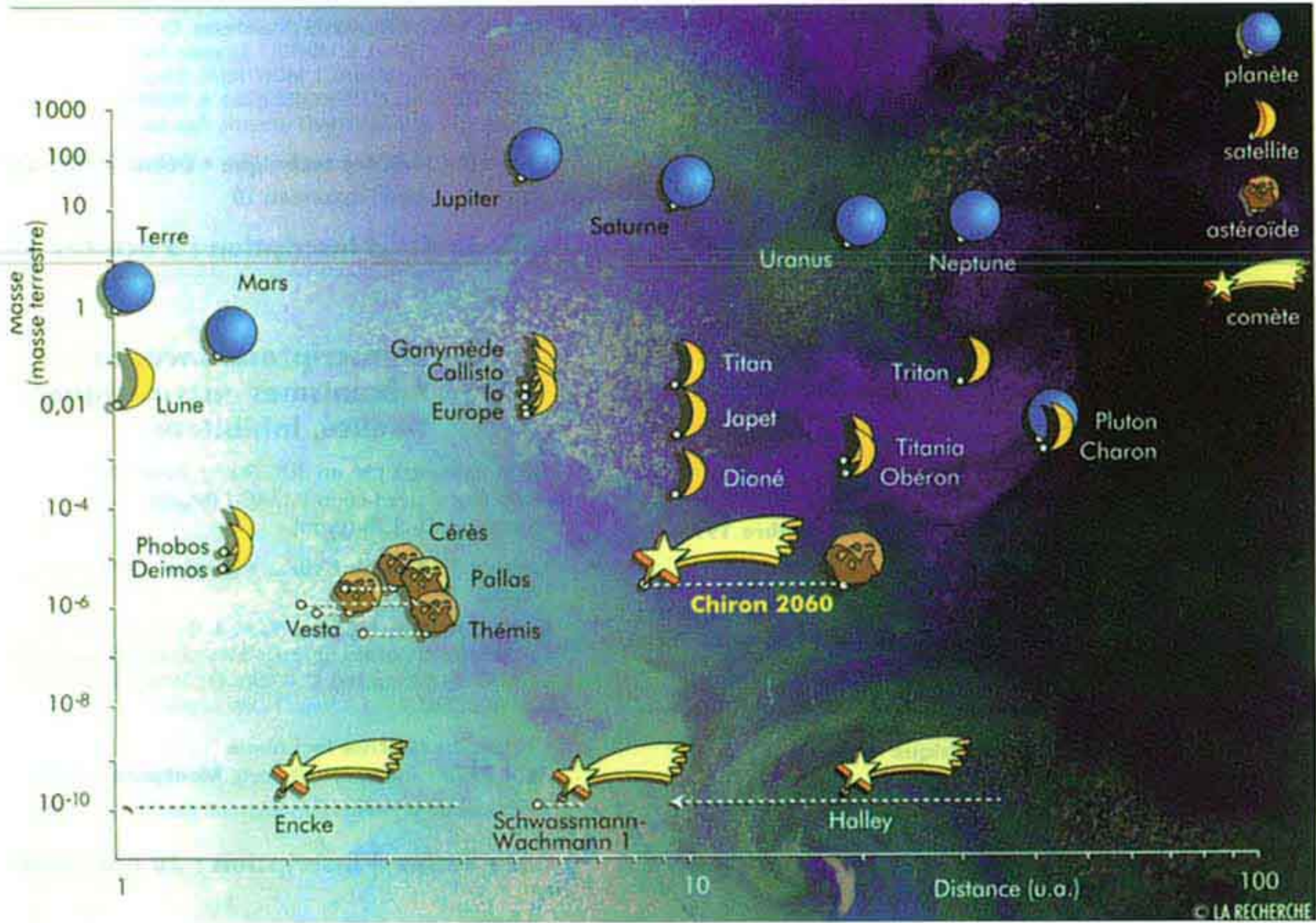
1. A. توزيع أفراد المجموعة الشمسية وفق العلاقة بين الكتلة منسوبة إلى كتلة الأرض Masse Terrestre والمسافة الفلكية A. منسوبة إلى بعد الأرض عن الشمس (150 مليون كم)
