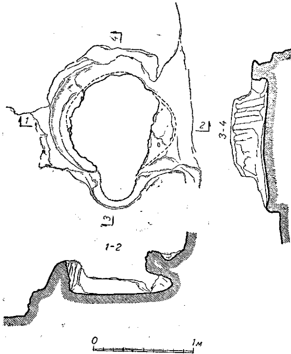
Рис. 5. План та розрізи глинобитної печі з житла XII—XIII ст.
