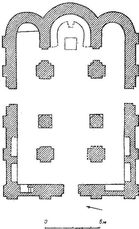
Рис. 24. Руїни шестистовпного храму XII ст. План.
