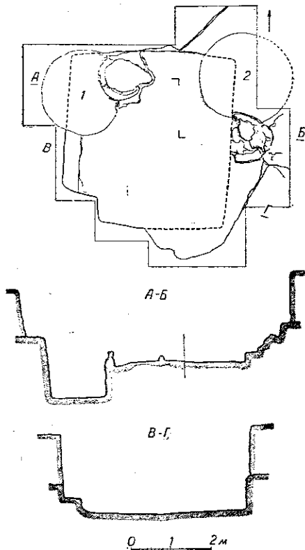
Рис. 4. Переяслав-Хмельницький. План та розріз жител XII—XIII ст. Розкопки 1952 р.
