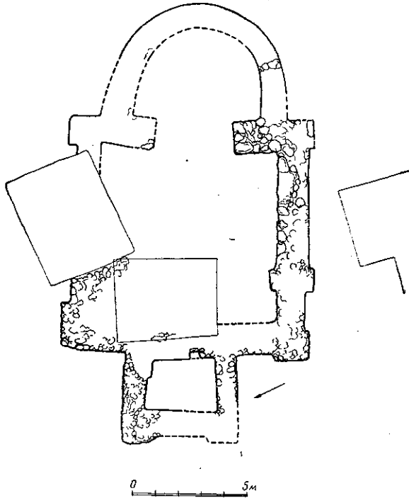
Рис. 1. Переяслав-Хмельницький. План руїн одноапсидного храму XI ст. Розкопки 1952 р.
