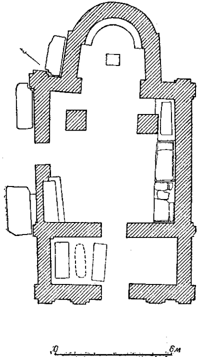
Рис. 17. Храм-усипальня XI ст. План.
