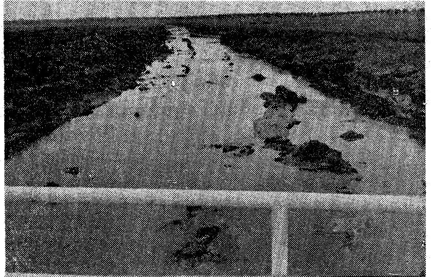
El Guadiana a su paso por las tierras debatidas. Las máquinas excavadoras han ampliado el cauce a unas aguas de irregular curso que producen encharcamientos en unos terrenos que se consideran aprovechables agrícolamente. Foto GARCIA de MORA.
