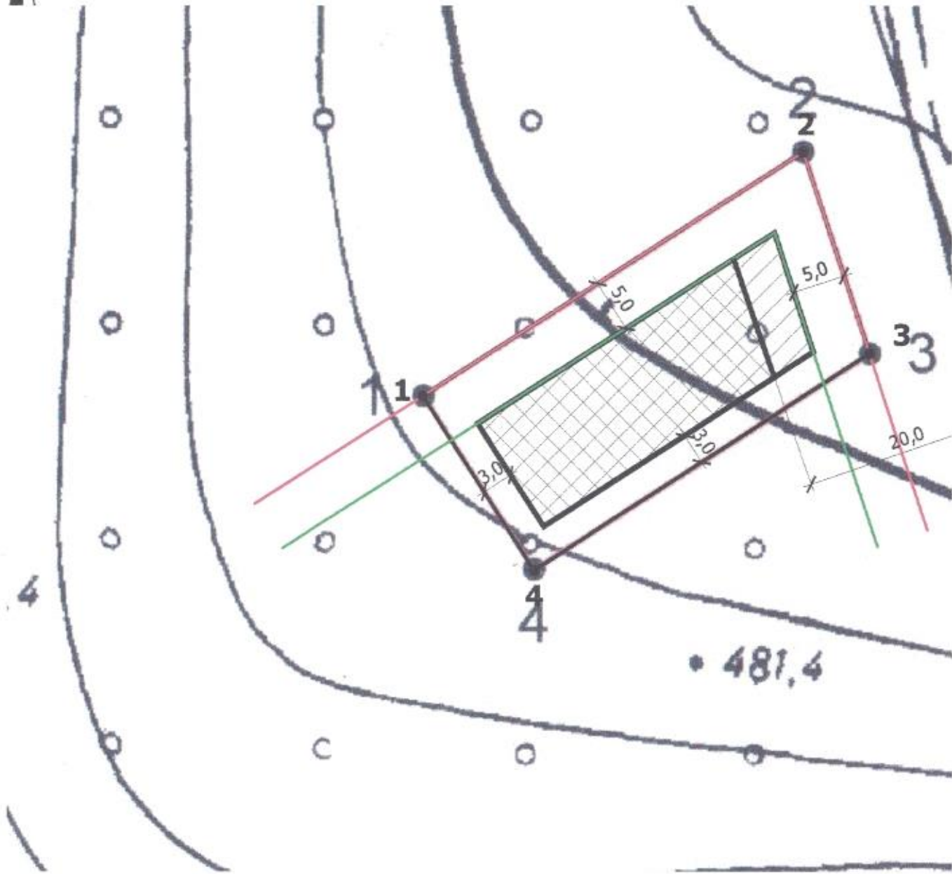
Ситуационный план
