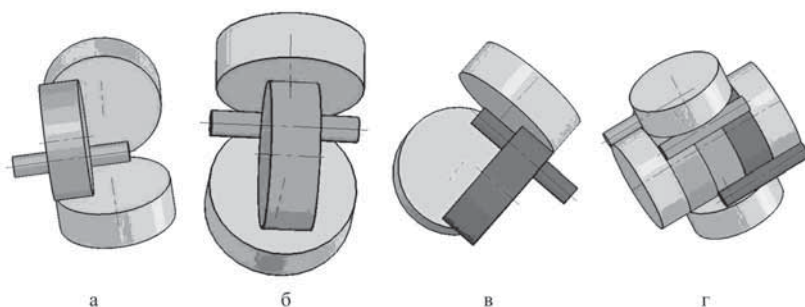
Рис. 2. Три конформации МЛП (а-в), способствующие созданию кубической (г) конформации элементарной липопептидной частицы (ЭЛПЧ).
