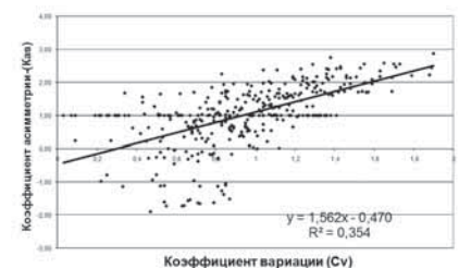
Рис.3. Взаимосвязь коэффициента асимметрии и вариации
