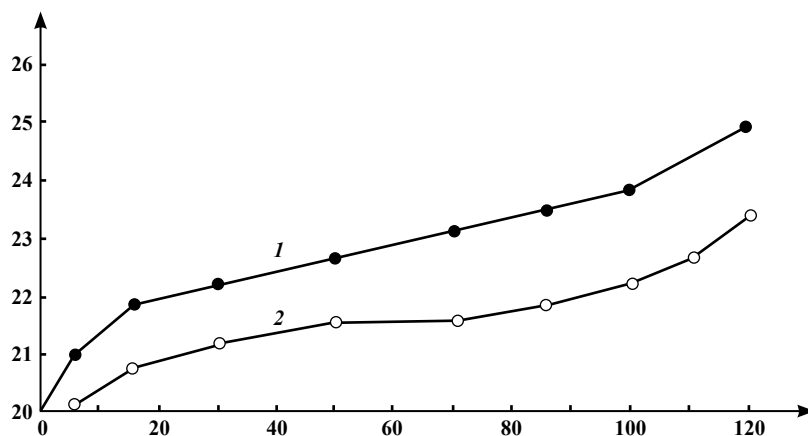
Рис. 1. Динамика повышения температуры поверхности мыши в зависимости от облучения: 1 – при мощности дозы 1,62 мкЗв/час; 2 – при мощности дозы 0,163 мкЗв/час.
