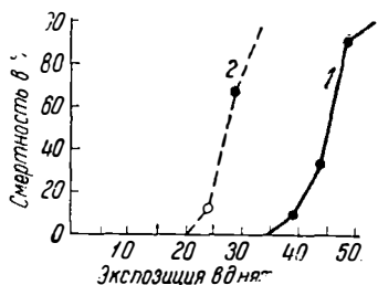
Рис. 3. Смертность зимующих жуков песчаного медляка ( Opatrum sabulosum L.) при различных экспозициях: 1 — при -7^{\circ} ; 2 — при -11^{\circ} .
