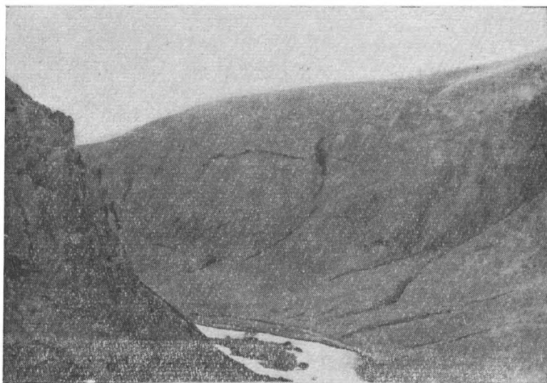
Фиг. 3. Каньон р. Раздан. Слева — четвертичные базальты, справа — мергели бозбурунской свиты.
