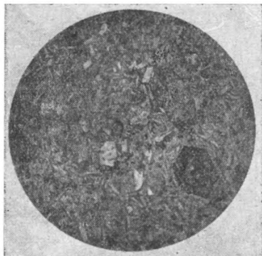
Фиг. 30. Обр. 237/50. d поля зрения 2,3 мм, без анализатора. Роговообманковый андезит. Порфирировая структура с микролитовой основной массой.
