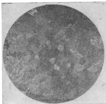
Фиг. 5б. Обр. 254а/51. d поля зрения 2,3 мм, николи скрещены. Известняк. Участок мозаичной структуры, сложенный доломитом (?).
