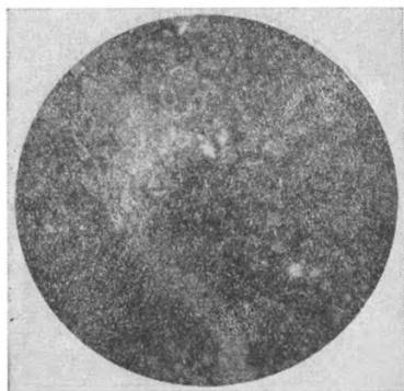
Фиг. 44. Обр. 154/51. d поля зрения 2,3 мм, без анализатора. Мергелевидный известняк. Органогенно-пелитовая структура.
