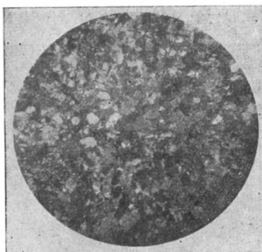
Фиг. 16. Обр. 105/50. d поля зрения 2,3 мм, николи скрещены. Сильно известковистая, сильно песчанистая глина. Пелитоалевритовая структура. Часть песчаных и алевритовых зерен представлена карбонатом.
