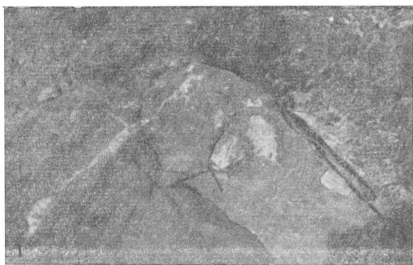
Фиг. 27. Крупнообломочная брекчия метаморфических сланцев в мергелях бжнинского разреза айриджинского горизонта (уменьшено примерно в 30 раз).
