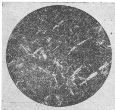
Фиг. 50 1 . Обр. XX/51. d поля зрения 2,3 мм, николи скрещены.
