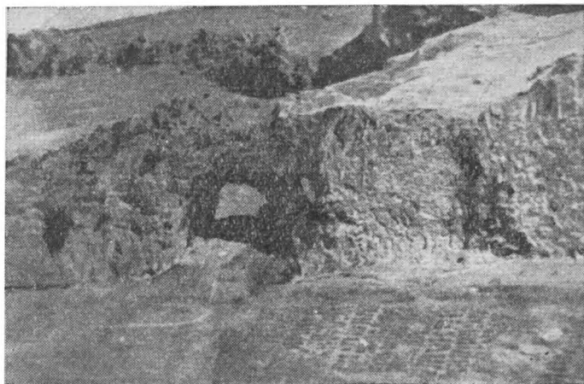
Фиг. 2. Золотые ворота в стене базальтов на левом берегу р. Раздан между селениями Бжни и Арзакан.
