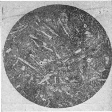
Фиг. 10 1 . Обр. 283/51. d поля зрения 2,3 мм, николи скрещены. Диабаз. Микродиабазовая структура.
