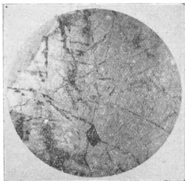
Фиг. 50. Обр. XX/51. d поля зрения 2,3 мм, без анализатора.
