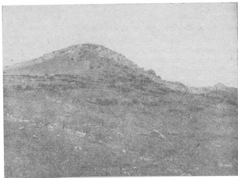
Фиг. 25. Мощная пачка песчаников и конгломератов азизкендского горизонта в верхнем течении р. Кесуз.
