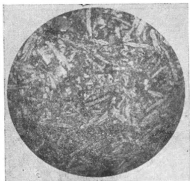
Фиг. 38. Обр. 181/51. d поля зрения 2,3 мм, без анализатора. Спилит. Интерсертальная (апоинтерсертальная) структура.
