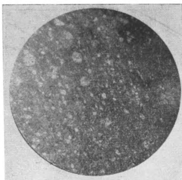
Фиг. 28. Обр. 205/50. d поля зрения 2,3 мм, без анализатора. Мергель. Пелитовая (мергельная) структура. Неяснослоистая текстура.
