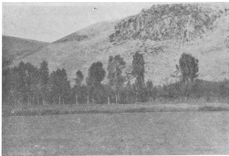
Фиг. 1. Левобережный пойменный остров р. Раздан между селениями Бжни и Арзакан.
