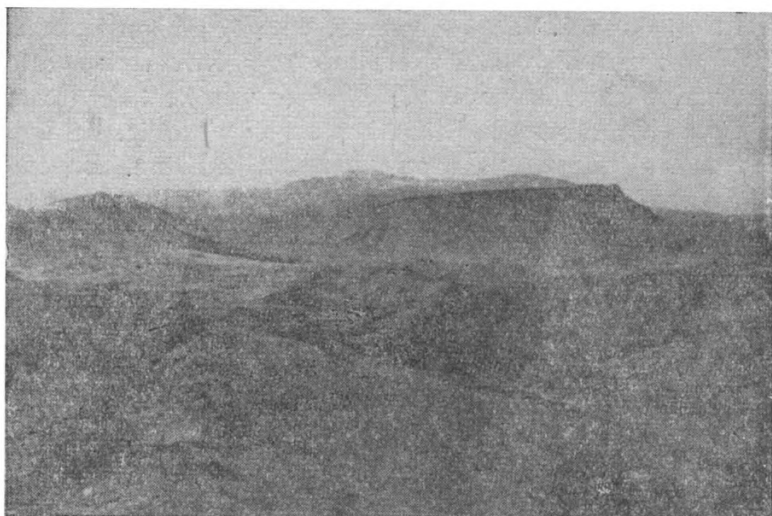
Фиг. 16. „Дурные земли“ Подкетузского участка.
