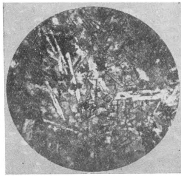
Фиг. 37 1 . Обр. 172/51. d поля зрения 0,7 мм, без анализатора. Мандельштейновый порфирит. Феррографическая структура базиса.
