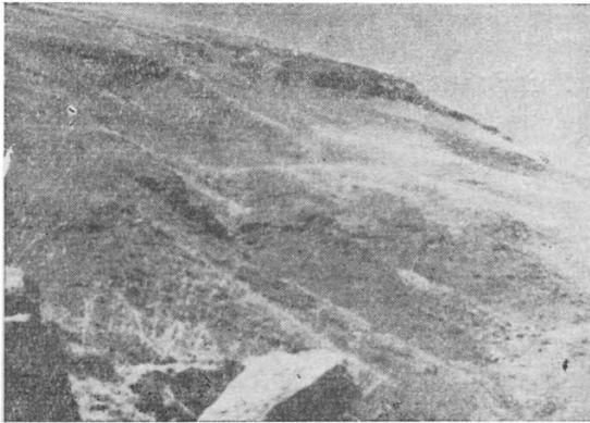
Фиг. 9. Выходы верхнего мела агверанского разреза.
