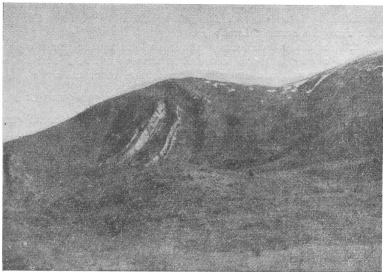
Фиг. 23. Пласты известняков ахсуинского горизонта на крутопадающем восточном крыле Ахсуинской антиклинали.
