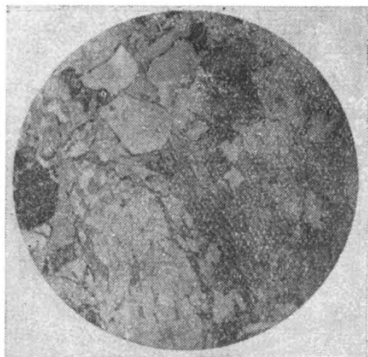
Фиг. 17. Обр. 107/50. d поля зрения 2,3 мм, без анализатора. Слабо глинистый, слабо известковистый песчаник. Крупнозернистая псаммитовая структура. Среди зерен кварца и полевых шпатов часты (середины нижней части шлифа) крупные обломки слюд (сланцевых сланцев).
