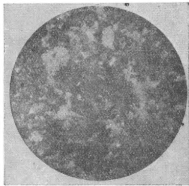
Фиг. 22. Обр. 110/50. d поля зрения 2,3 мм, без анализатора. Амфиболит. Гранобластовая структура (обломок брекчии).
