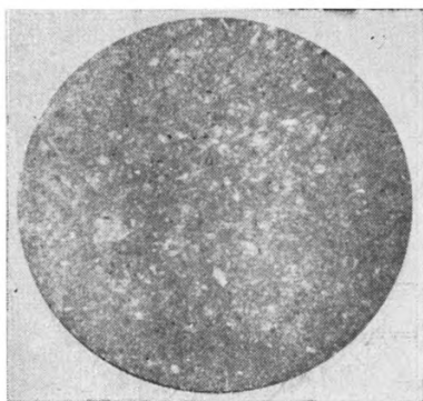
Фиг. 40. Обр. 190/51. d поля зрения 2,3 мм, без анализатора. Субалевритовый высококарбонатный мергель. Пелитовая (мергельная) структура с участками алевропелитовой.
