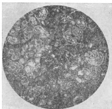
Фиг. 8. Обр. 266/51. d поля зрения 2,3 мм, без анализатора. Высококарбонатный мергель. Органогенная (микроракушечниковая) структура.
