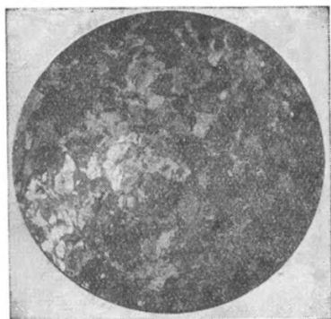
Фиг. 49. Обр. Д3/51. d поля зрения 2,3 мм, без анализатора. Измененное роговообманковое габбро. Субгранобластовая структура.
