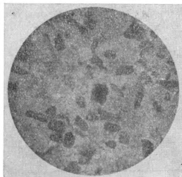
Фиг. 45. Обр. 155/51. d поля зрения 2,3 мм, без анализатора. Известняк. Органогенно-гранобластовая структура с реликтовыми участками глинистой массы.
