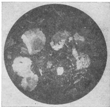
Фиг. 36а 1 . Обр. 302/51. d поля зрения 4,1 мм, николи скрещены.
