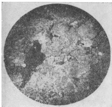
Фиг. 5а. Обр. 254а/51. d поля зрения 2,3 мм, без анализатора. Известняк. Крупнозернистая гранобластовая мраморовидная структура. Участки клетчатого строения являются, возможно, не реликтами растительных тканей, как указано в тексте, а остатками раковин верхнемелового рода Lepidorbitoides Silvestri.
