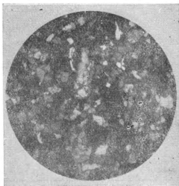
Фиг. 2. Обр. 237/51, d поля зрения 2,3 мм, николи скрещены. Сильно глинистый алевролитовый, мелкозернистый песчаник. Алевропсаммитовая структура.
