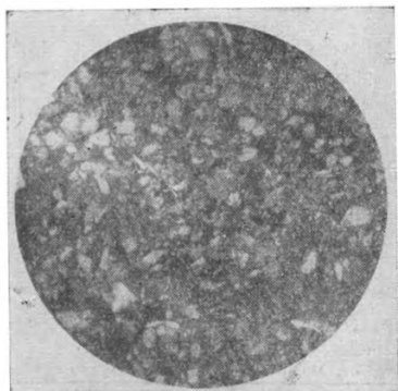
Фиг. 1. Обр. 231/51. d поля зрения 2,3 мм, без анализатора. Сильно песчанистая, алевролитовая глина. Алевропелитовая структура с участками псаммоалевритовой
