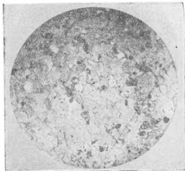
Фиг. 20. Обр. 123/50. d поля зрения 2,3 мм, без анализатора. Мергель. Микрогранобластовая структура, с редкими раковинами фораминифер (аномалина—справа внизу).
