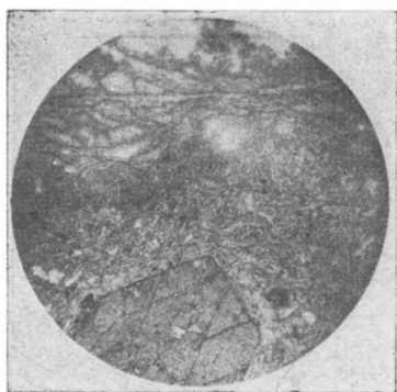
Фиг. 31. Обр. 207 2 /50. d поля зрения 2,3 мм, без анализатора. Роговообманковый андезит. Крупнопорфирировая структура с микролитовой основной массой. В верхней части шлифа сплошная полоса мраморизованного карбоната мергелей (образец шлифа взят в контакте андезита и мергелей).
