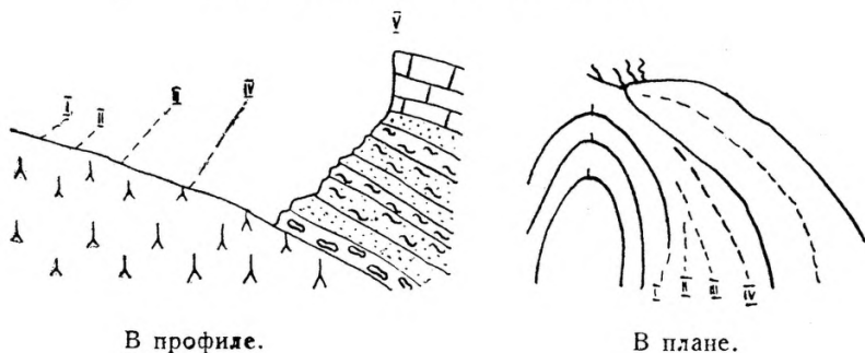
Схема развития „скользящих“ долин
