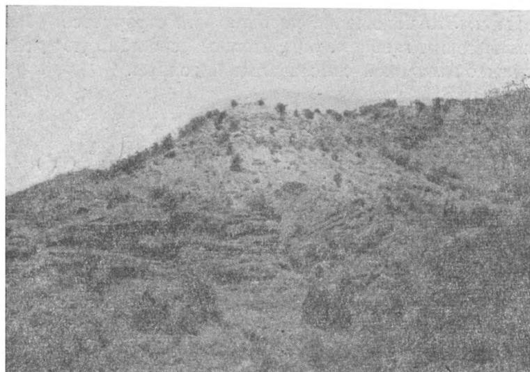
Фиг. 18. Мощный пласт крупновалунных базальных конгломератов в основании азизкендского горизонта, залегающих на порфиритах хосровской толщи в среднем течении р. Хосров.
