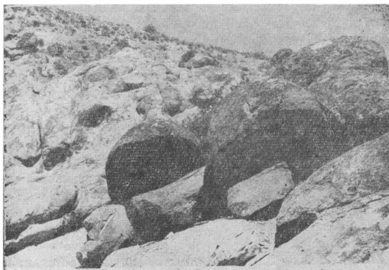
Фиг. 8. Андезитовые шары-в Малой бозбурунской котловине.
