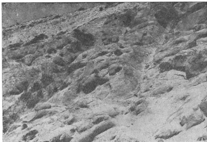
Фиг. 7. Шаровая (концентрически-скорлуповатая) отдельность андезитов Бозбурунского лакколита. Малая (южная) котловина.
