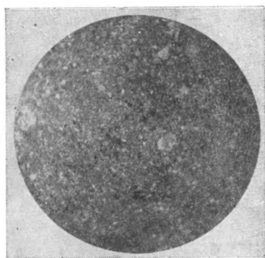
Фиг. 43. Обр. 206/51. d поля зрения 2,3 мм, без анализатора. Доломитистый мергель (?). Пелитовая (мергельная) структура с участками алевропелитовой.
