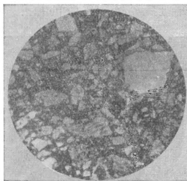
Фиг. 4. Обр. 234/51. d поля зрения 2,3 мм, без анализатора.
