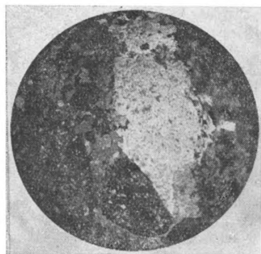
Фиг. 15 1 . Обр. 296/51. d поля зрения 2,3 мм, николи скрещены. Карбонатный силицит. Скрытокристаллическая структура. На просветленном участке раскристаллизованный кремнезем загрязнен некремнистыми частицами.
