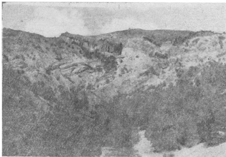
Фиг. 19. Несогласное налегание эоценовых песчаников (верхний карниз) на породы бозбурунской свиты в верхнем течении р. Хосров.
