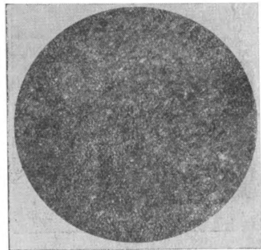
Фиг. 13. Обр. 75/51. d поля зрения 2,3 мм, без анализатора. Мергель. Пелитовая (мергельная) структура.
