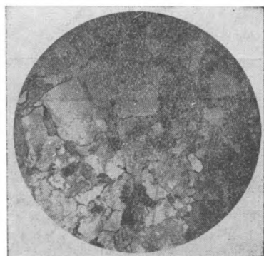
Фиг. 3. Обр. 233/51. d поля зрения 2,3 мм, без анализатора.
