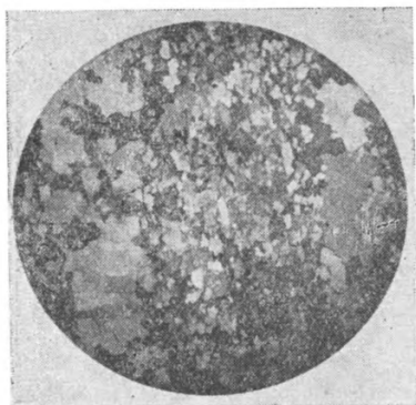
Фиг. 25. Обр. 16/50. d поля зрения 2,3 мм, николи скрещены. Слюдистый кварц-полевошпатовый сланец. Микрогранобластовая структура с удлиненными взаимопараллельными участками гранобластовой (субмозаичной).
