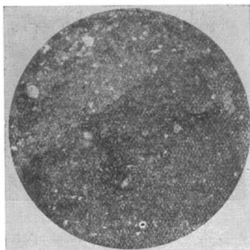
Фиг. 7. Обр. 272/51. d поля зрения 2,8 мм, без анализатора. Мергель, пелитовая (мергельная) структура с редкими раковинами фораминифер.
