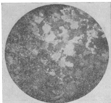
Фиг. 24. Обр. 1ж/50. d поля зрения 2,3 мм, николи скрещены. Слюдистый кварц-полевошпатовый сланец. Микрогранобластовая структура с удлиненными участками гранобластовой (субмозаичной).
