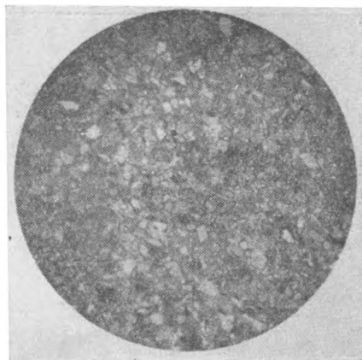
Фиг. 34. Обр. 325/51. d поля зрения 2,3 мм, без анализатора. Слабо песчаный алевритовый известняк. Мелкозернистая псаммитовая структура с участками алевритовой.
