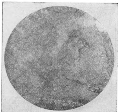
Фиг. 48. Обр. Д1/51. d поля зрения 2,3 мм, без анализатора. Роговообманковое габбро (габбро-амфиболит?). Крупнозернистая габбровая структура. Четко выделяется шагреневая поверхность амфиболов, занимающих большую часть шлифа.
