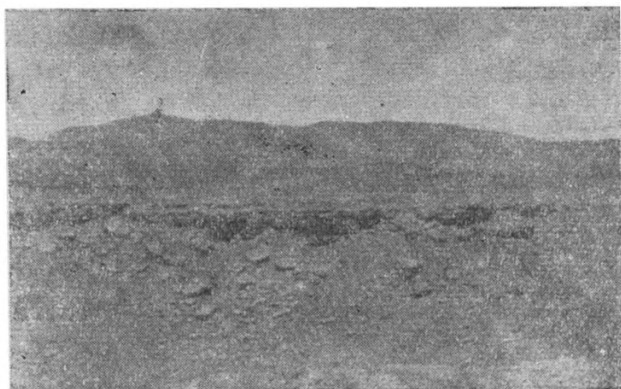
Фиг. 15. Один из травертиновых покровов в районе сел. Дашлу.
