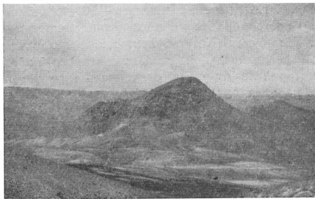
Фиг. 6. Обнажение андезитов Иландагского нечка.
