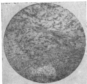
Фиг. 26. Обр. 1в/50. d поля зрения 2,3 мм, без анализатора. Слюдистый (слюдяной) сланец. Гранолепидобластовая структура. Четко выделяются вытянутые включения слюд.
