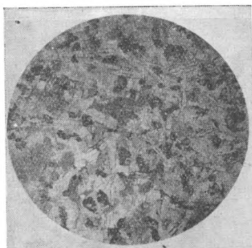
Фиг. 9. Обр. 64/51. d поля зрения 2,3 мм, без анализатора. Диабаз. Микродиабазовая структура.
