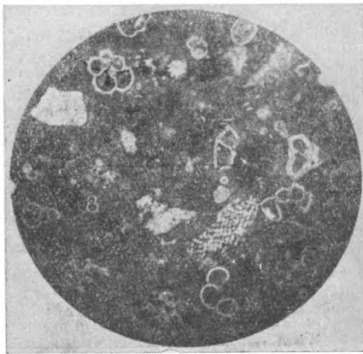
Фиг. 12. Обр. 275/51. d поля зрения 2,3 мм, без анализатора. Высококарбонатный мергель. Органогенно-пелитовая структура. Хорошо видны срезы конических глоботрункан. Участок клетчатого строения, возможно, является остатком раковины лепидорбитондеса.
