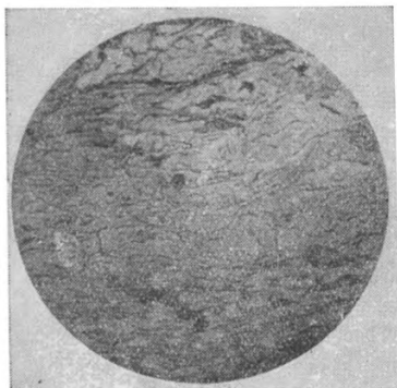
Фиг. 23. Обр. 1 д/50. d поля зрения 2,3 мм, без анализатора. Амфиболит. Микрогранобластовая сублепидобластовая структура. Бросается в глаза высокий шагреньевый рельеф почти всей поверхности шлифа.
