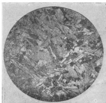
Фиг. 10. Обр. 283/51. d поля зрения 2,3 мм, без анализатора. Диабаз. Микродиабазовая структура.
