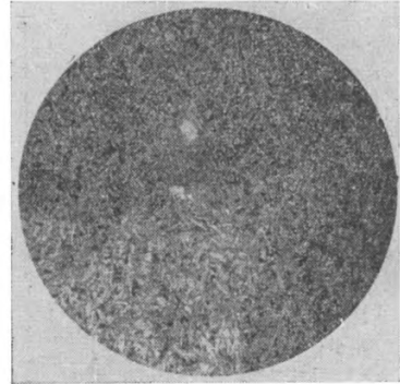
Фиг. 11. Обр. 284/51. d поля зрения 2,3 мм, без анализатора. Диабаз. Микродиабазовая (субмикродиабазовая) структура. Участок в центре шлифа заполнен хлоритом и кальцитом,
