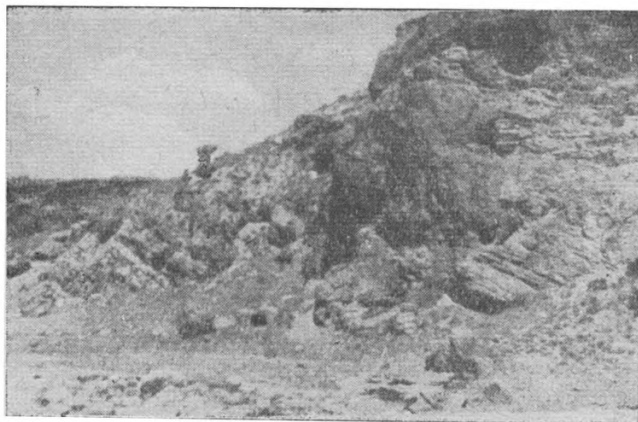
Фиг. 14. Налегание горизонтально, залегающих травертинов на дислоцированные мергели бозбурунской свиты в Котурбулагской долине.
