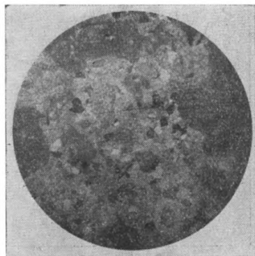
Фиг. 42. Обр. 200/51. d поля зрения 2,3 мм, без анализатора. Псаммитовый высококарбонатный мергель. Псаммоалевритовая структура с участками карбонатно-глинистой (мергельной) массы (по краям).
