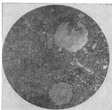
Фиг. 39. Обр. 303/51. d поля зрения 4,1 мм, без анализатора. Манделштейновый порфирит (манделштейн). Миндалекаменная (манделштейновая) текстура, спилитовая, частью интерсертальная структура.
