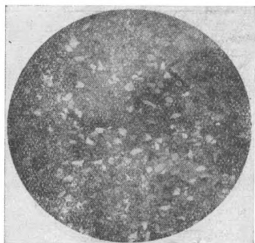
Фиг. 46. Обр. 164/51. d поля зрения 2,3 мм, николи скрещены. Конгломератовый известняк (цемент). Алевропелитовая структура. За пределами поля зрения на отдельных участках развита гранобластовая структура с реликтами глинистой массы.
