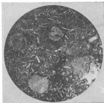
Фиг. 37. Обр. 172/51. d поля зрения 4,1 мм, без анализатора. Мандельштейновый порфирит (мандельштейн). Миндалекаменная текстура, сплитовая структура.
