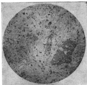
Фиг. 32. Обр. 219/50. d поля зрения 2,3 мм, без анализатора. Роговообманковый андезит. Порфирировая структура с микролитовой основной массой. На фоне микролитов плагиоклаза и стекла четко выделяются темные микролиты роговой обманки.
