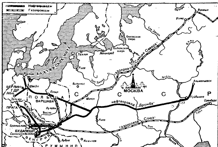
Схема нефте- и газопроводов
