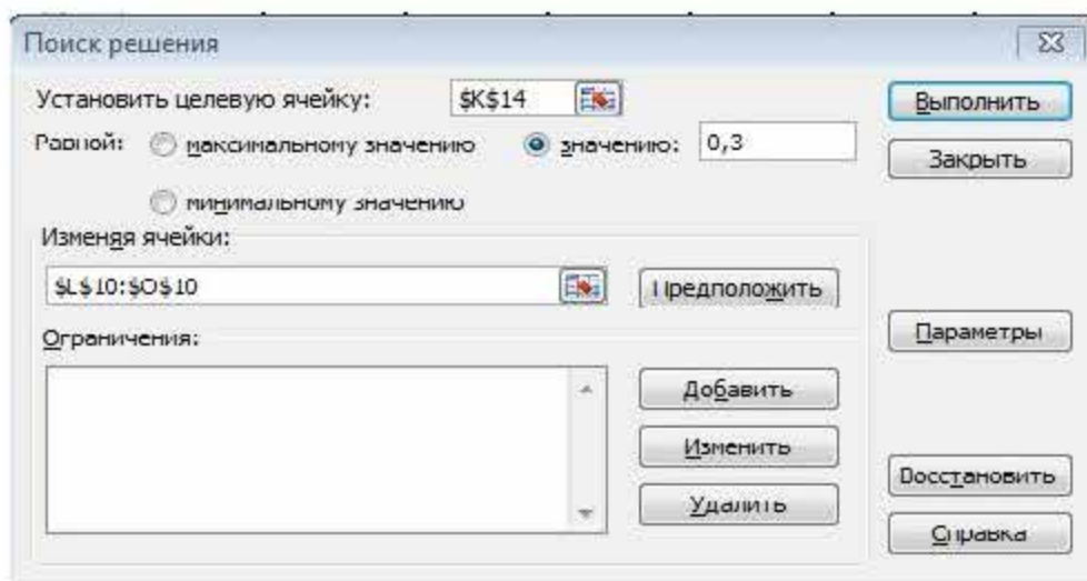
Рис. 5.12. Діалогове вікно «Поиск решения» для оптимізації інтегрального показника*
