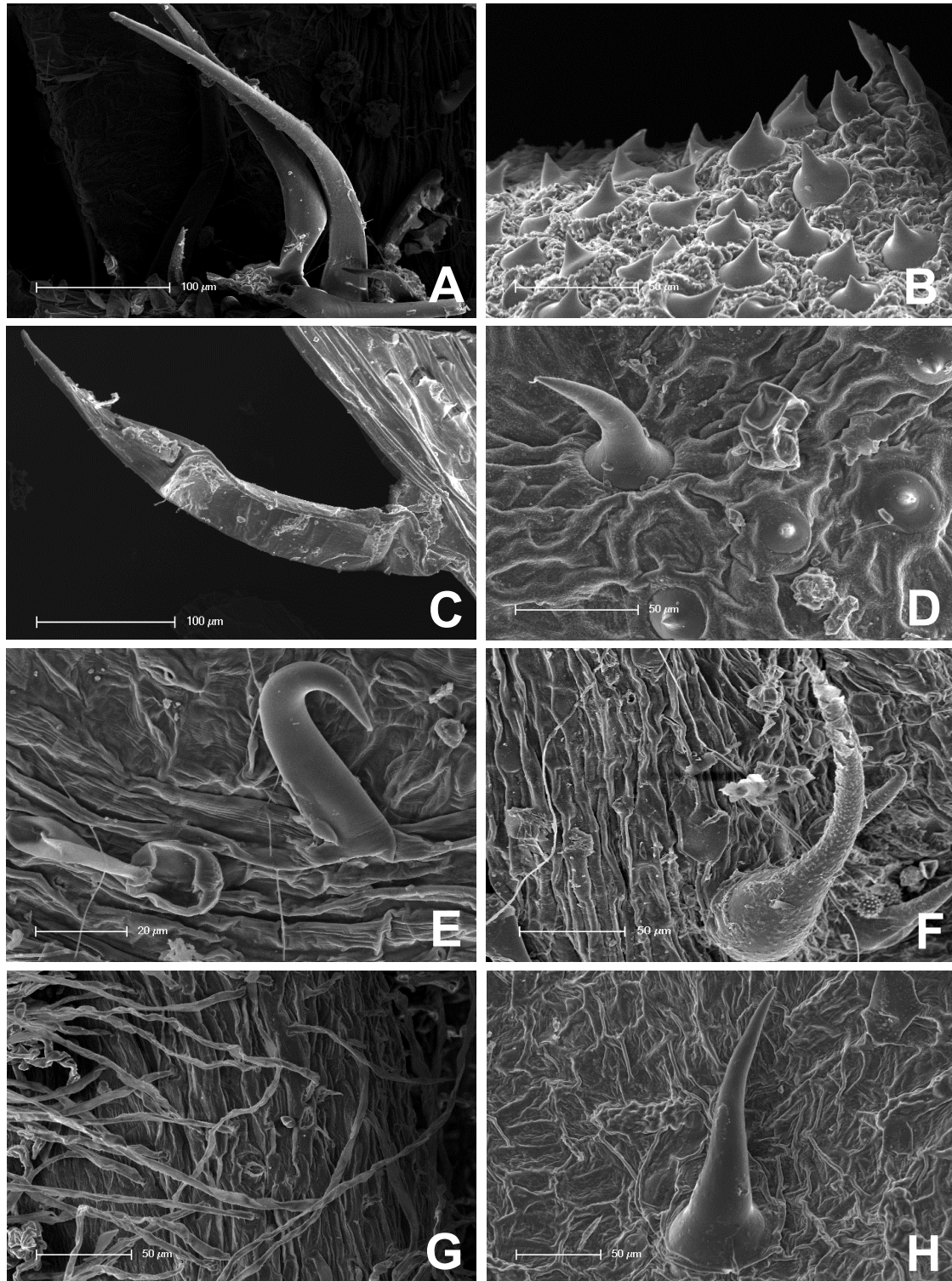
Figura 3. A. Boehmeria caudata , tricomas simples longo e cilíndrico, próximo à base do perigônio da flor pistilada; B. Cecropia hololeuca , tricomas simples curtos, na porção mediana do perigônio da flor pistilada; C. Pilea hyalina , tricoma simples e pluricelular, próximo à inserção do pecíolo na lâmina; D. Cecropia pachytachya , tricoma simples curto e cônico, na face adaxial foliar próximo à margem; E. Boehmeria caudata , tricomas simples uncinado e liso, na face adaxial foliar próximo à margem; F. Boehmeria cylindrica , tricoma simples longo e verrugoso, na face abaxial foliar próximo ao ápice; G. Cecropia glaziovii , tricomas simples, unicelulares, plissados e entrelaçados, na face abaxial foliar próximo à margem; H. Ureia caracasana , tricoma glandular urente e cystólitos fusiformes, face abaxial foliar próximo à nervura central. (A: Bertani 17; B: Romaniuc Neto 761; C: Gehrt s.n., SP 4020; D: Romaniuc Neto 1364; E: Loefgren 235; F: Mattos 9150; G: Romaniuc Neto 760; H: Barreto 3472).
