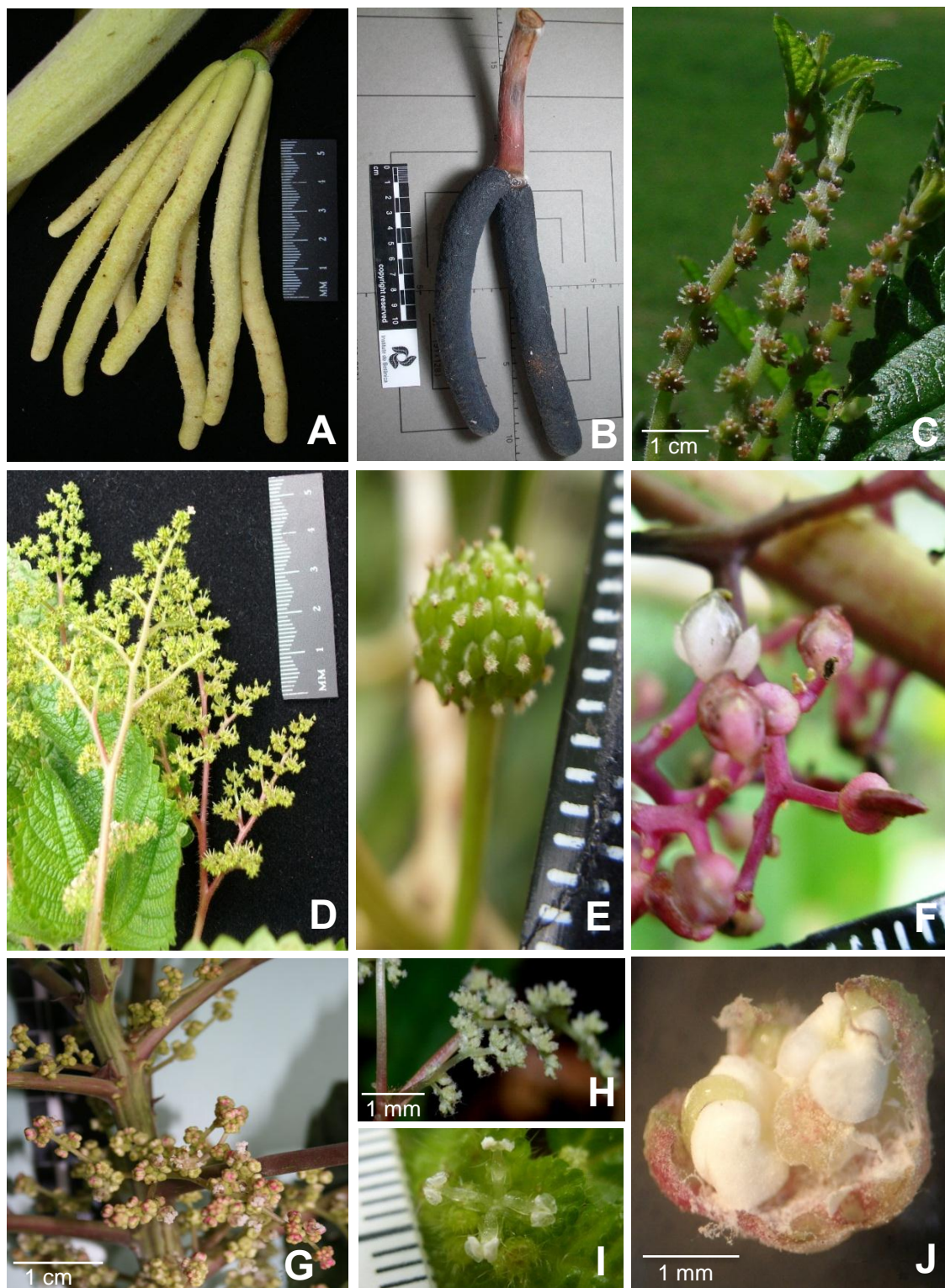
Figura 5. Variação das inflorescências e flores em Urticaceae. A. Cecropia pachystachya , Amento estaminado. B. Cecropia hololeuca , Amento pistilado. C. Boehmeria cylindrica , Inflorescência em glomérulos. D. Laportea aestuans , Inflorescência em panícula. E. Coussapoa microcarpa , Inflorescência pistilada em capítulo. F. Urera nitida , Inflorescência pistilada em cimeira dicotômica. G. Urera baccifera , Inflorescência estaminada em cimeira escorpióide. H. Pilea pubescens , Inflorescência em fascículo. I. Pilea pubescens , Flor estaminada. J. Urera baccifera , Corte longitudinal do botão estaminado, estames inflexos. (Fotos de André Luiz Gaglioti: A, B, C, D, E, F, G, H, J. Foto de Leandro Cardoso Pederneiras: I). Régua milimetrada: E, F, I.
