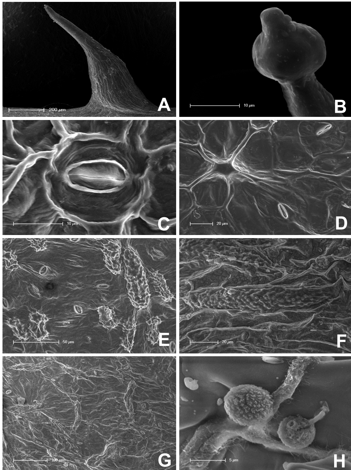
Figura 4. A. Urera nitida , tricoma glandular urente, na nervura central da face abaxial foliar; B. Urera baccifera , ápice do tricoma glandular urente do eixo da inflorescência pistilada; C. Phenax sonneratii , estômato paracítico, na face abaxial foliar, próximo à nervura central; D. Pilea rhizobola , cystólito puntiforme e estômatos, face abaxial foliar, próximo à nervura central; E. Urera baccifera , cystólitos fusiformes e estômatos, na face abaxial foliar, próximo à nervura central; F. Pilea microphylla , cystólitos lineares, na face adaxial; G. Pilea hyalina , cystólitos em forma de V aberto, na face abaxial foliar, próximo à nervura central; H. Pourouma guianensis , grãos de pólen. (A: Gaglioti 90; B: Gaglioti 93; C: Sendulsky 652; D: Edwall s.n. SP12781, E: Gaglioti 93; F: Gaglioti 87; G: Gehrt s.n., SP 4020; H: Furlan 1037).
