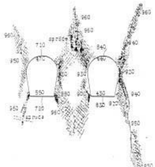
5. ábra: Károsodási mintázat, mely egy egytengelyű nyomófeszültségnek kitett dupla vágat körül alakul ki (túlterhelés hatására) [Leon és Willheim 1914c].
