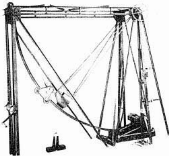
20. ábra A Charpy által javasolt 200 mkp-os ütőmű
