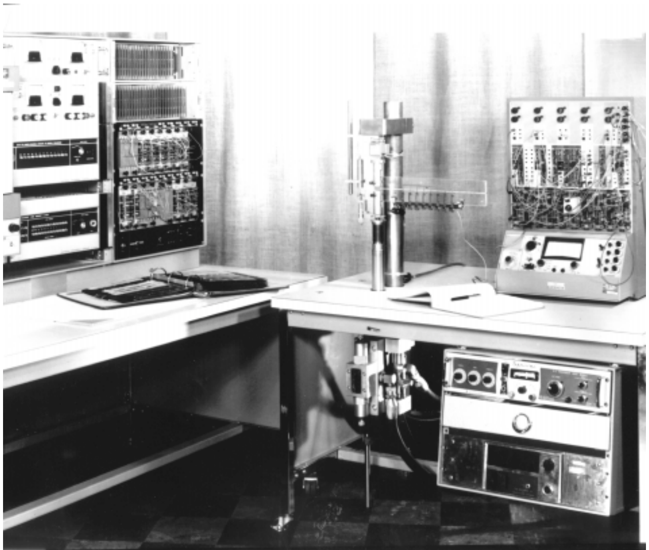
28. ábra. George IRWIN laboratóriumában elkészített első, analóg számítógép vezérelte anyagvizsgáló berendezés (1964)
