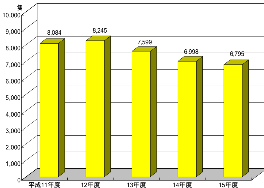
小樽港 入港船舶数の推移
