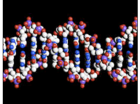
DNA.
