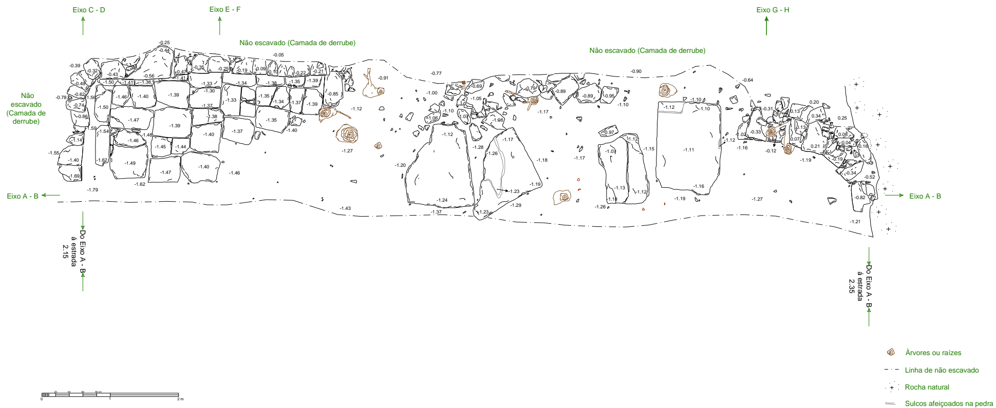
Planta geral do balneário este [ver ficheiro original ]
