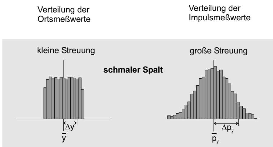
Abbildung 7.13: Verteilung der Orts- und Impulsmesswerte für einen schmalen Einzelspalt
