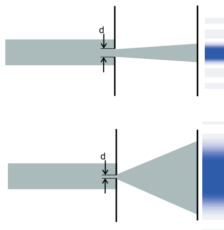
Abbildung 7.11: Elektronen am Einzelspalt
