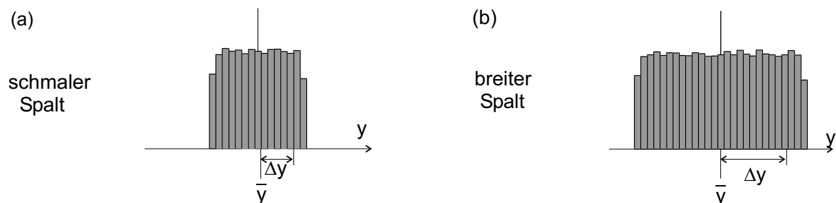
Abbildung 7.5: Verteilung der Ortsmesswerte bei verschiedenen Spalten
