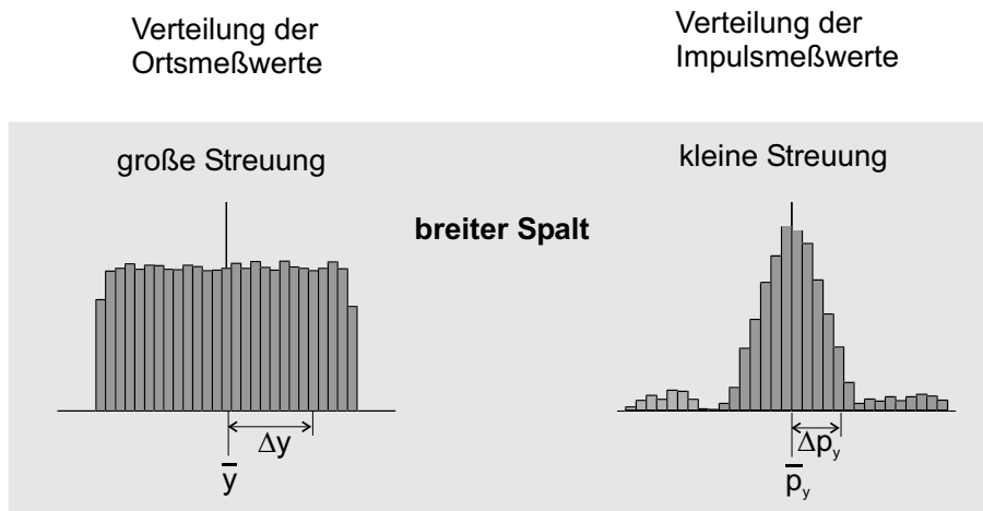
Abbildung 7.12: Verteilung der Orts- und Impulsmesswerte für einen breiten Einzelspalt
