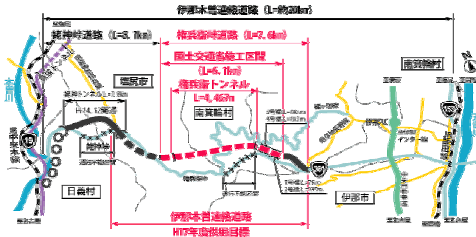
図 1-1 伊那木曾連絡道路の概要図
