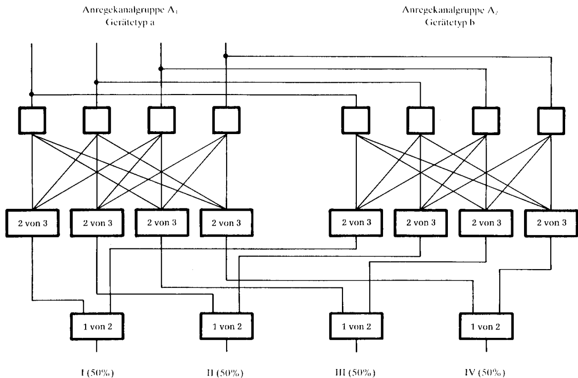
Bild 4-8: Für die Auslösung von 4 zueinander redundanten 50%-Sicherheitssteleinrichtungen bei einem Störfall, für dessen Erkennung nur eine einzige Sicherheitsvariable vorhanden ist, ist der hier dargestellte prinzipielle Schaltungsaufbau möglich, wenn Folgeausfälle im Bereich der Meßwerterfassung (z. B. Bruch einer Wirkdruckleitung) physikalisch möglich und nicht auslösegerichtet zu unterstellen sind. Die Geräte zur Meßwerterfassung bis einschließlich Meßumformer in den beiden Meßkanalgruppen sind diversitär (Gerätetyp a und Gerätetyp b).
