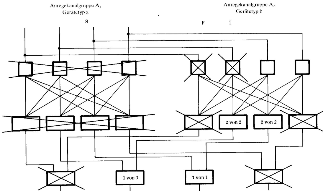
Bild 4-9: Bei ungünstigster Ausfallkombination kann aus dem System nach Bild 4-8 folgendes entstehen: Während der Instandsetzung eines Anregelkanals in Anregelkanalgruppe A tritt ein systematischer Geräteausfall im Gerätetyp a auf. Zusätzlich wird ein Anregelkanal in der Anregelkanalgruppe A 2 aufgrund eines Folgeausfalls funktionsunfähig. Der Störfall wird durch Auslösung von zwei 50%-Systemen ausreichend beherrscht.
