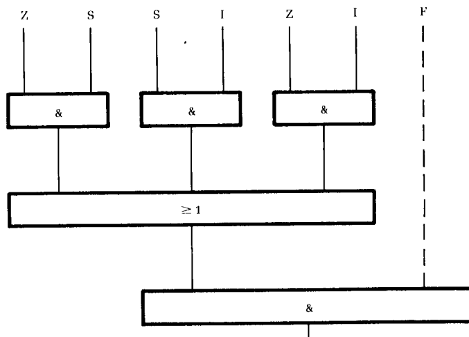
Bild 4-1: Anzuwendende Ausfallkombinationen
