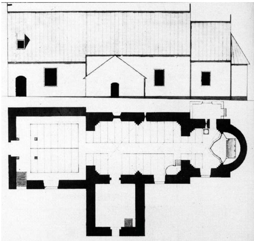
Denna planritning och fasad åt söder är uppgjord av murmästare S. Österberg år 1836 inför den planerade ombyggnaden.
