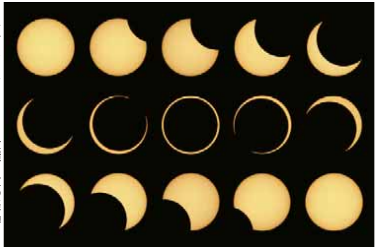
スペイン・マドリッド金環日食の経過
