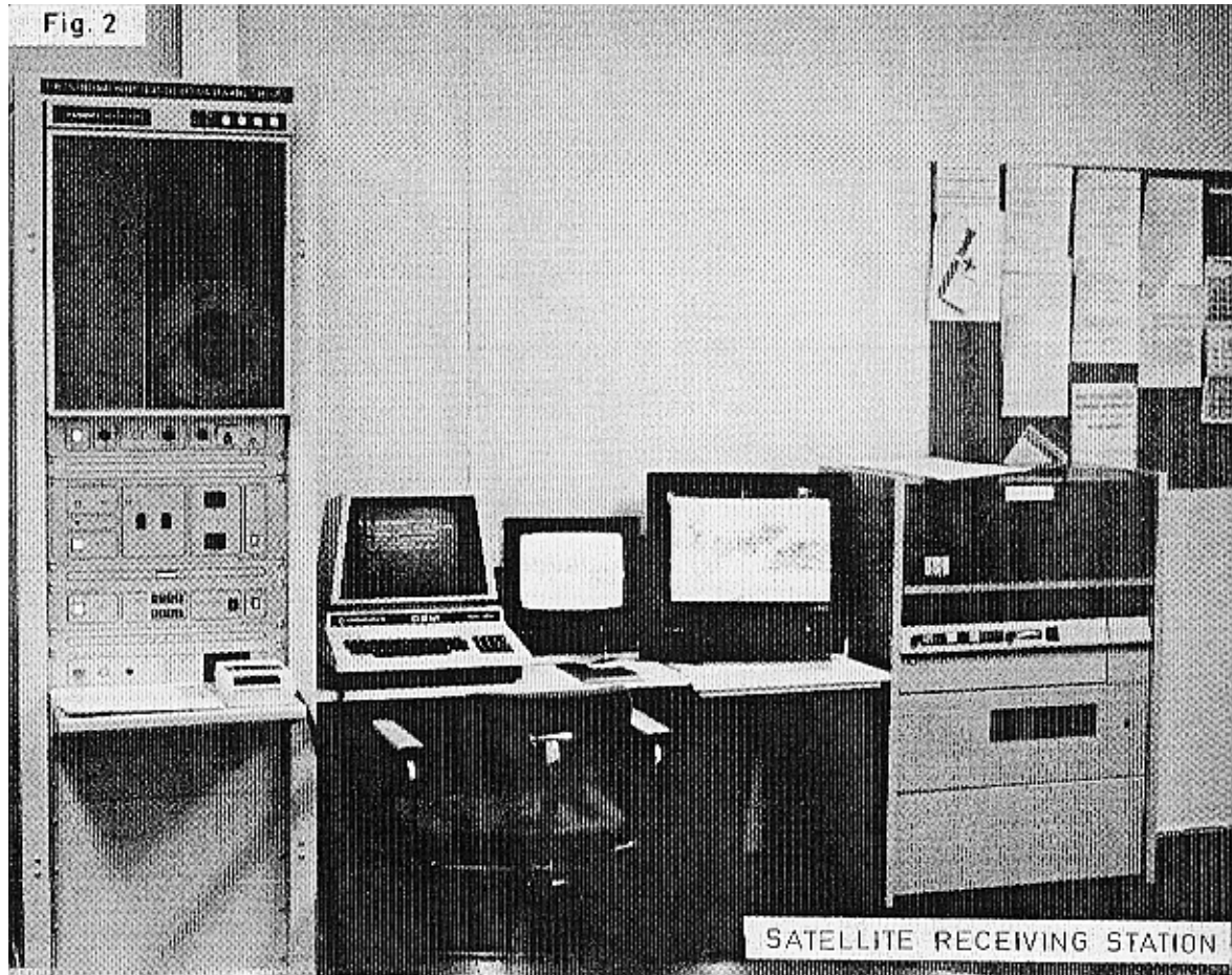
Kuva 48. NOAA-kuvien vastaanottolaitteisto. Vasemmalla ohjausyksikkö ja instrumenttinauhuri, rataennusteiden laskuun käytetty tietokone, kaksi monitoria ja äärimmäisenä oikealla kuvapiirturi.
