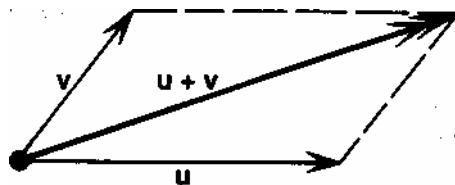
FIGURA V.6. Ley del paralelogramo para la suma vectorial.
