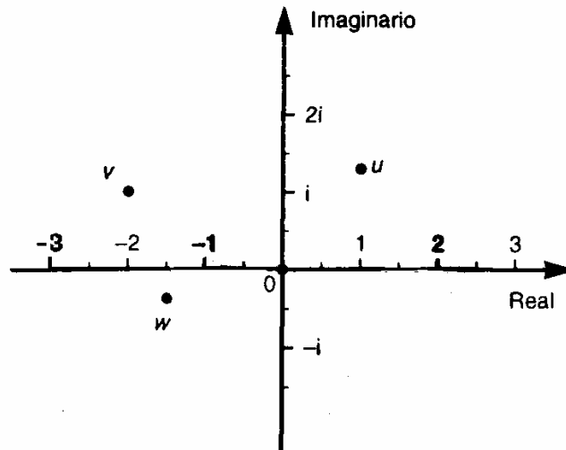
FIGURA III.9. Localizaciones en el plano de Argand de u=1+i1.3 , v=-2+i y w=-1.5-i0.4
