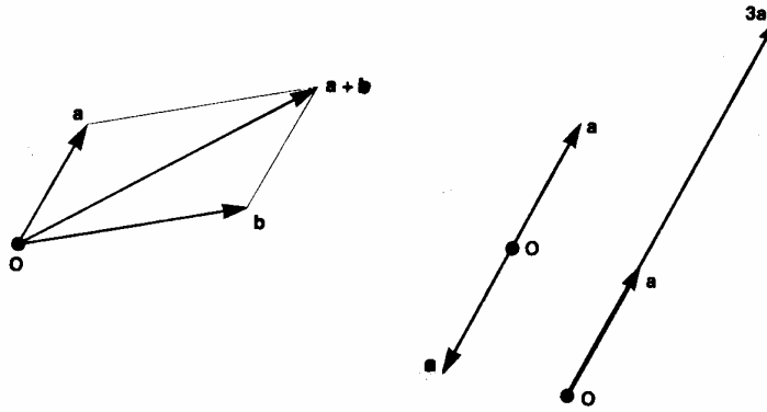
FIGURA VI. 19. La suma de vectores en el espacio de Hilbert y la multiplicación por escalares pueden representarse normalmente, como en el caso de los vectores en el espacio ordinario.
