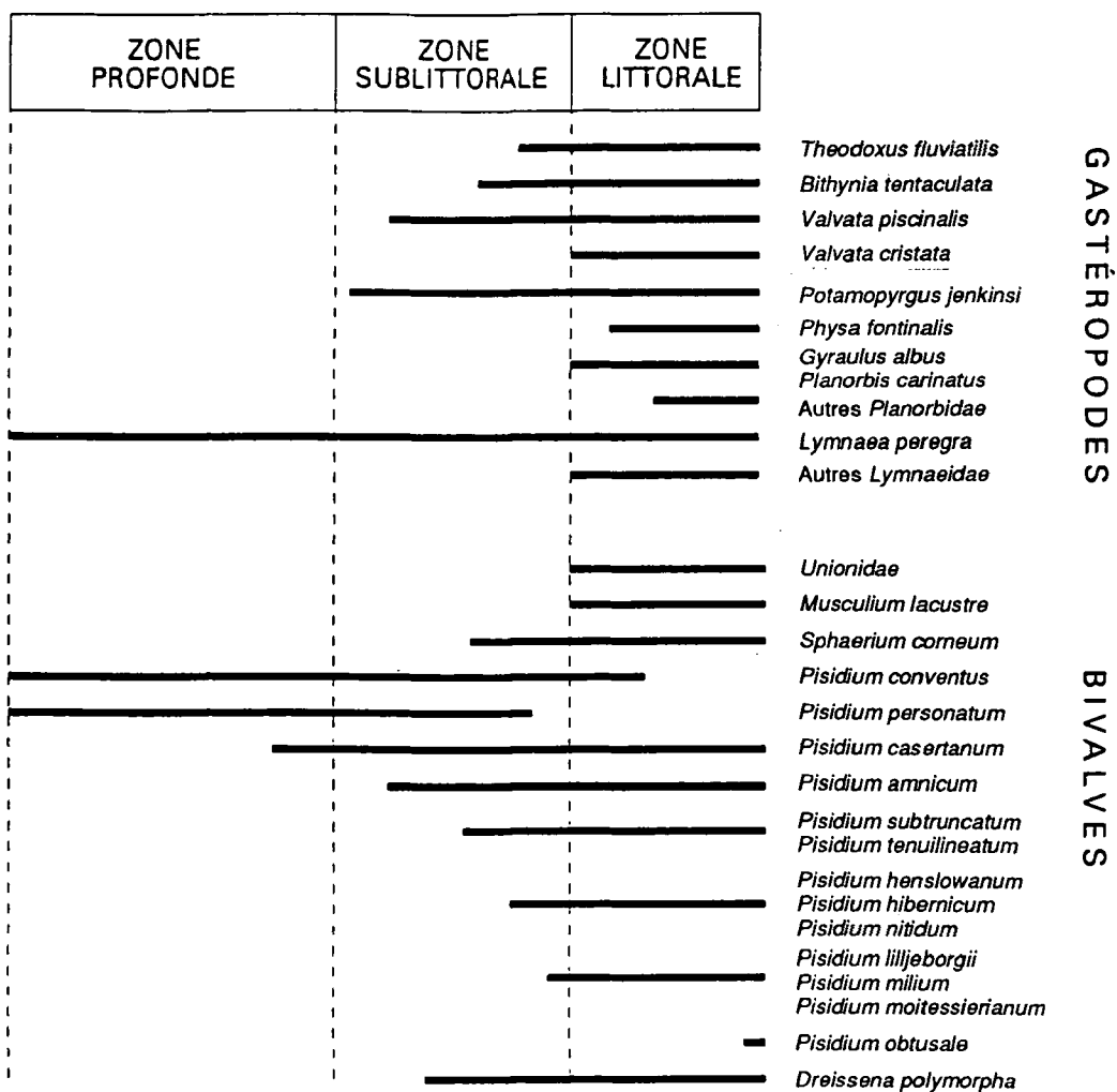
Figure 1 : Distribution bathymétrique des principales espèces de Mollusques dans un système lacustre théorique (d'après FAVRE 1927, 1940 ; CROZET, 1982 ; MOUTHON, 1987a ; MOUTHON & KUIPER, 1987c).
