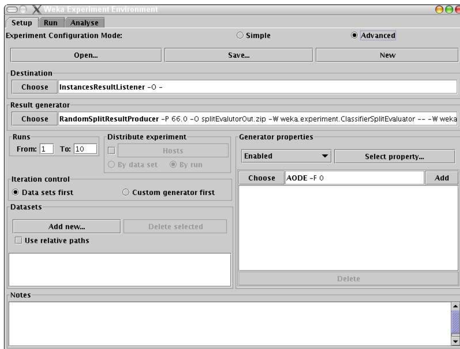
Figura 22: El modo experimentador, modo Advanced .
