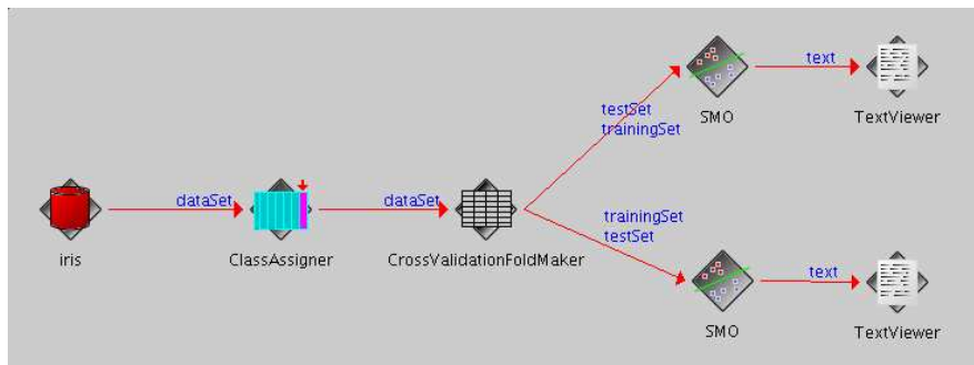
Figura 31: El experimento ya está completo.
