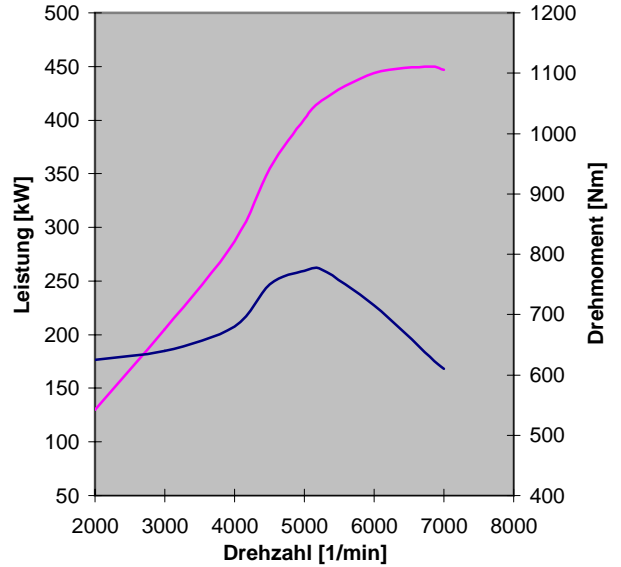
— Leistung — Drehmoment
